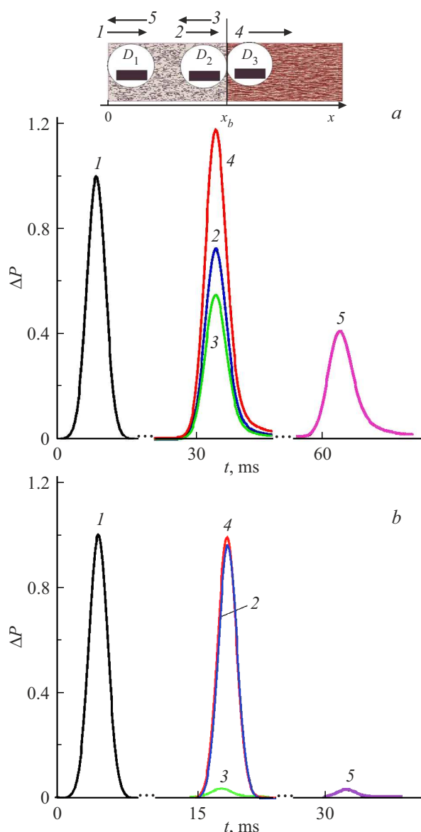
Рис. 4. Отражение и прохождение импульса „медленной“ (a) и „быстрой“ (b) волн границы между слоями ( \alpha_{g0} = 0.01 ). x_b = 5 (a) и 40 m (b). На вставке сверху — схема задачи: датчики D_1 , D_2 , D_3 расположены соответственно на границе расчетной области x = 0 , слева и справа от границы x = x_b . Цифры соответствуют расчетным осциллограммам: 1 — первоначальный импульс, 2 — импульс, распространяющийся слева направо на границе x = x_b , 3 — отраженный импульс, 4 — прошедший импульс, 5 — отраженный импульс, дошедший до границы x = 0 .
