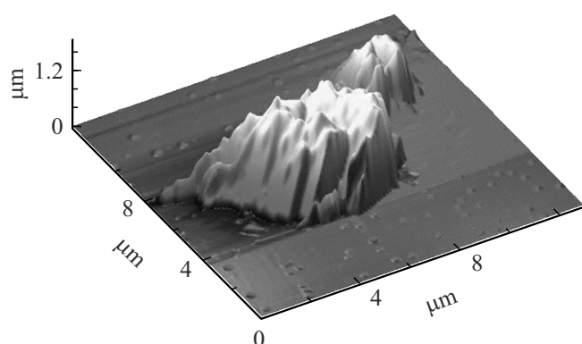
Рис. 3. Трехмерное АСМ изображение агломерата частиц, расположенного в центре созданной тестовой структуры в виде креста.
