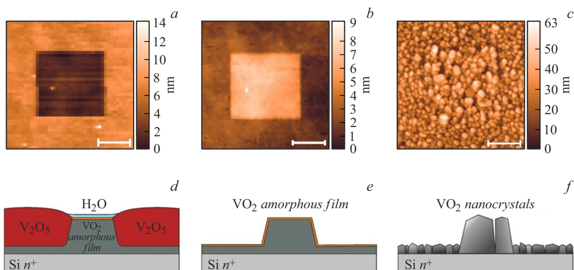
Рис. 5. АСМ изображения и схематические изображения этапов формирования нанокристаллов \text{VO}_2 различных размеров: a — формирование квадратной наноструктуры \text{VO}_2 методом о-СЗЛ; b — селективное удаление сформированного слоя \text{V}_2\text{O}_5 в воде; c — формирование кристаллических наноструктур \text{VO}_2 различных размеров в результате отжига; d — схематическое изображение a ; e — схематическое изображение b ; f — схематическое изображение c . Длина размерного отрезка — 500 нм.
