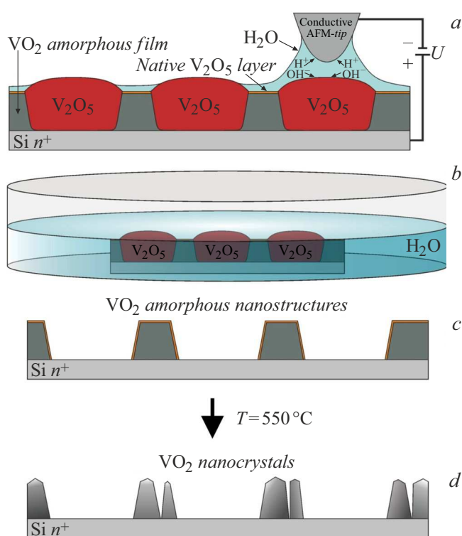
Рис. 4. Схематическое изображение формирования кристаллических наноструктур \text{VO}_2 : a — локальное окисление аморфной пленки \text{VO}_2 до \text{V}_2\text{O}_5 ; b — селективное удаление \text{V}_2\text{O}_5 в воде; c — сформированные аморфные наноструктуры \text{VO}_2 ; d — сформированные кристаллические наноструктуры \text{VO}_2 в результате отжига.
