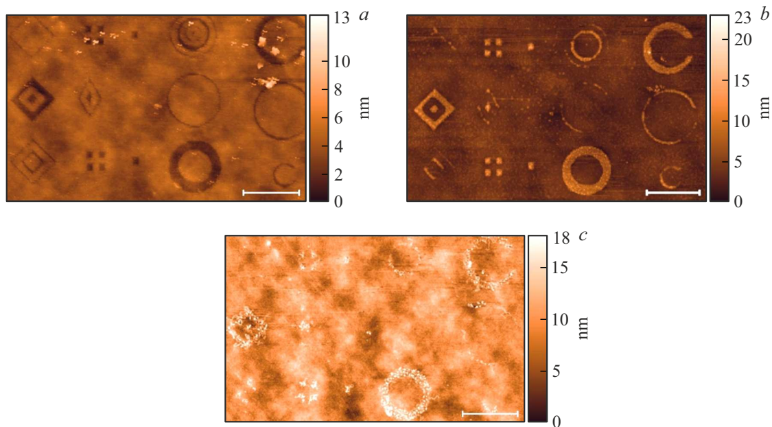
Рис. 7. АСМ изображения этапов формирования различных наноструктур \text{VO}_2 в виде ромбов, квадратов, колец и пр.: а — изображение поверхности после процедуры о-СЗЛ; b — изображение поверхности после удаления окисленного слоя \text{V}_2\text{O}_5 ; с — изображение поверхности после отжига и формирования кристаллических наноструктур \text{VO}_2 . Длина размерного отрезка — 1 \mu\text{m} .
