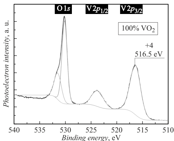
Рис. 1. Спектр РФЭС пленки \text{VO}_2 . Пик \text{V} 2p_{3/2} соответствует степени окисления ванадия +4.
