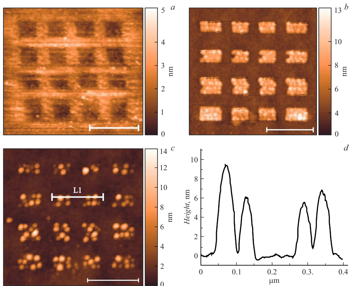
Рис. 2. АСМ изображения этапов формирования наноструктур \text{VO}_2 : a — окисление всей поверхности, кроме массива 4 \times 4 наноструктур; b — удаление сформированного \text{V}_2\text{O}_5 ; c — формирование нанокристаллов \text{VO}_2 после отжига; d — профиль вдоль линии L1 на рис. 2, c . Длина размерного отрезка — 400 nm.
