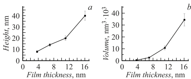
Рис. 6. Зависимости высоты (а) и объема (b) одиночных нанокристаллов \text{VO}_2 в формируемых наноструктурах \text{VO}_2 от толщины модифицируемой аморфной пленки \text{VO}_2 .
