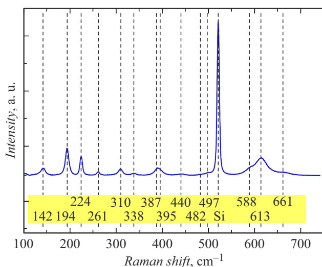
Рис. 3. Спектр КРС образца с кристаллическими наноструктурами \text{VO}_2 .
