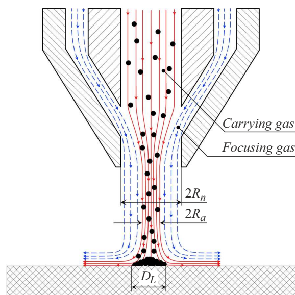
Рис. 1. Принципиальная схема фокусирующей системы аэрозольного принтера.
