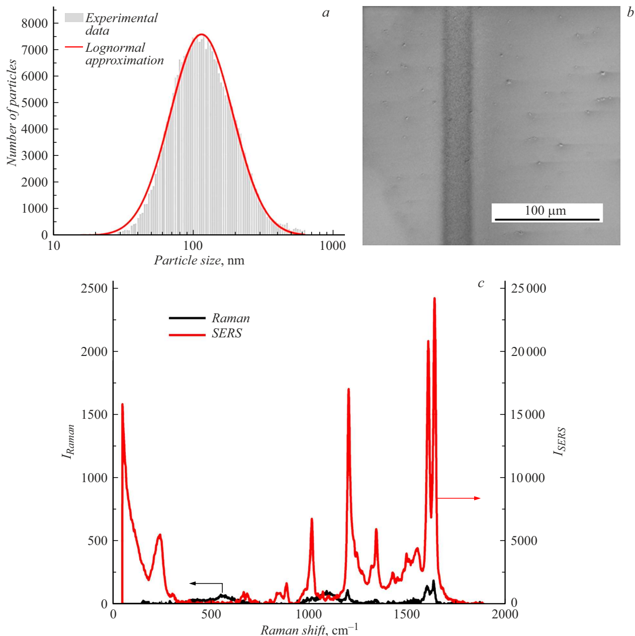
Рис. 2. a — распределение Au наночастиц по размерам на выходе из фокусирующего сопла; b — РЭМ изображение плазмонной наноструктуры в виде печатной линии; c — сопоставление спектров ВРЕ (1,2-бис(4-пиридил)этилена): красным обозначен SERS-спектр, полученный для раствора с концентрацией 10 -4 mol/l на печатной линии с высотой 0.1 μm, черным — исходный рамановский спектр для раствора концентрации 10 -2 mol/l.
