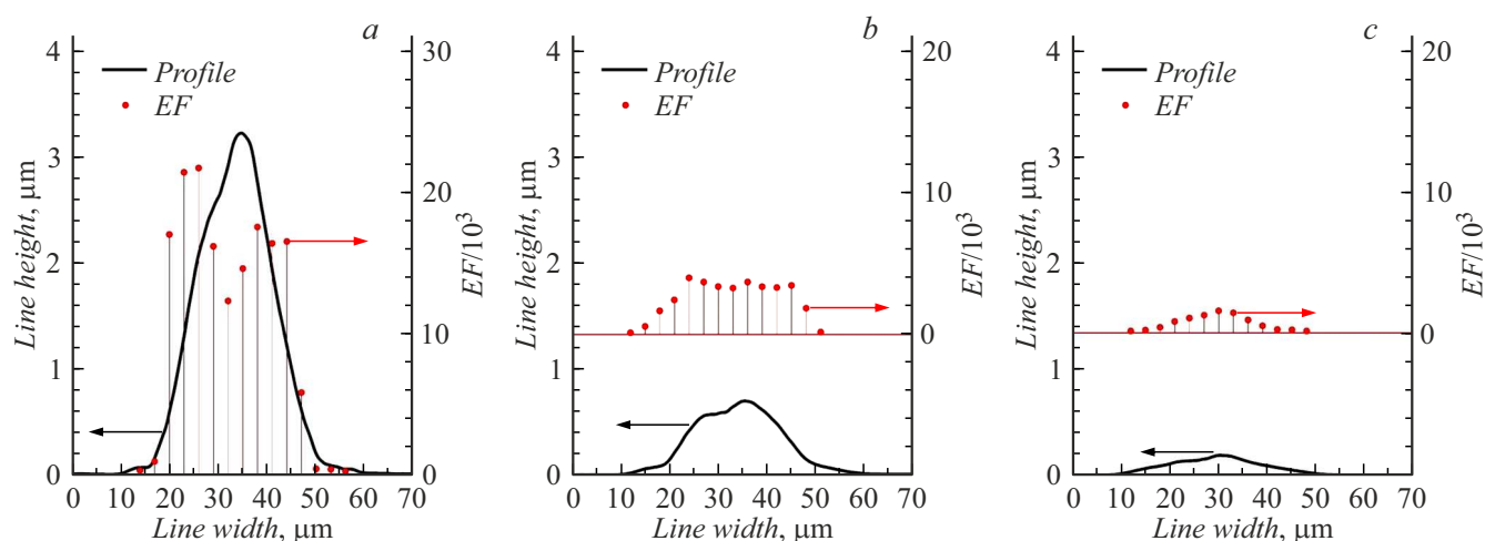
Рис. 3. Профили плазмонных наноструктур и значения коэффициента плазмонного усиления при толщине печатной линии 3.2 (a), 0.8 (b) и 0.2 μm (c).
