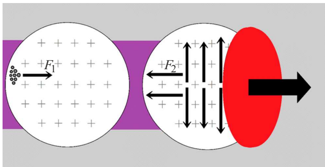
Рис. 2. Иллюстрация трехмерной модели, в которой фемтосекундный лазерный импульс порождает пондеромоторную силу F_2 , выталкивающую электроны из области высокой интенсивности лазерного поля, вследствие чего образуется ионная полость. F_1 обозначает силу, ускоряющую электронный пучок, захваченный внутри ионной полости.
