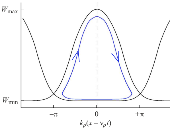
Рис. 4. Фазовая траектория захваченного в ионную плотность электронного пучка. Фазовые траектории частиц являются замкнутыми и находятся в области, ограниченной сепаратрисами. Покуда электроны находятся в области k_{pl}(x - v_{phase\ pl}t) < 0 , пучок ускоряется, а после прохождения точки 0 и приобретения максимальной энергии, не превышающей максимального теоретического значения W_{max} , начинается замедление.
