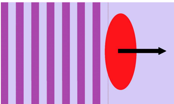
Рис. 1. Схематическая иллюстрация одномерной модели, в которой проходящий через плазму лазерный импульс возбуждает бегущую за ним ленгмюровскую волну с периодической модуляцией электронной плотности (волну сжатия и растяжения).
