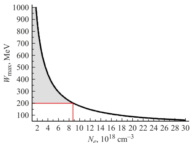
Рис. 5. Зависимость максимально возможного теоретического значения энергии ускоренного пучка W_{\max} от электронной плотности плазмы. Закрашенная область соответствует диапазону значений n_e , при которых W_{\max} > 200 MeV, а необходимая требуемая мощность фемтосекундной лазерной системы еще не превышает 100 TW.
