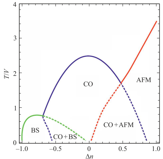
Рис. 6. Фазовая диаграмма модельного никелата при V = 1 , J = 1 , t = 1 , U = 0 . Пунктир — границы областей фазового расслоения CO+BS и CO+AFM.
