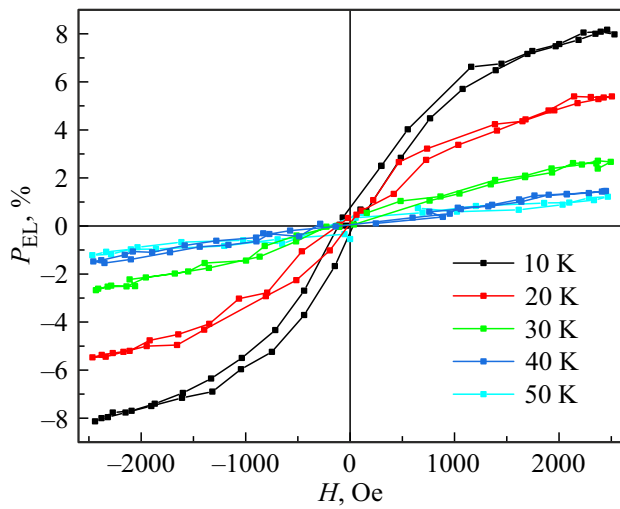
Рис. 3. Магнитооптические зависимости степени циркулярной поляризации P_{EL}(H) для Образца 2, измеренные в диапазоне температур 10–50 К.
