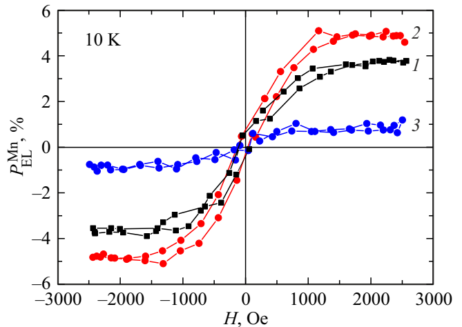
Рис. 4. Магнитооптические зависимости степени циркулярной поляризации P_{EL}^{Mn}(H) для исследуемых образцов, измеренные при температуре 10 К. Номера кривых соответствуют номерам образцов.
