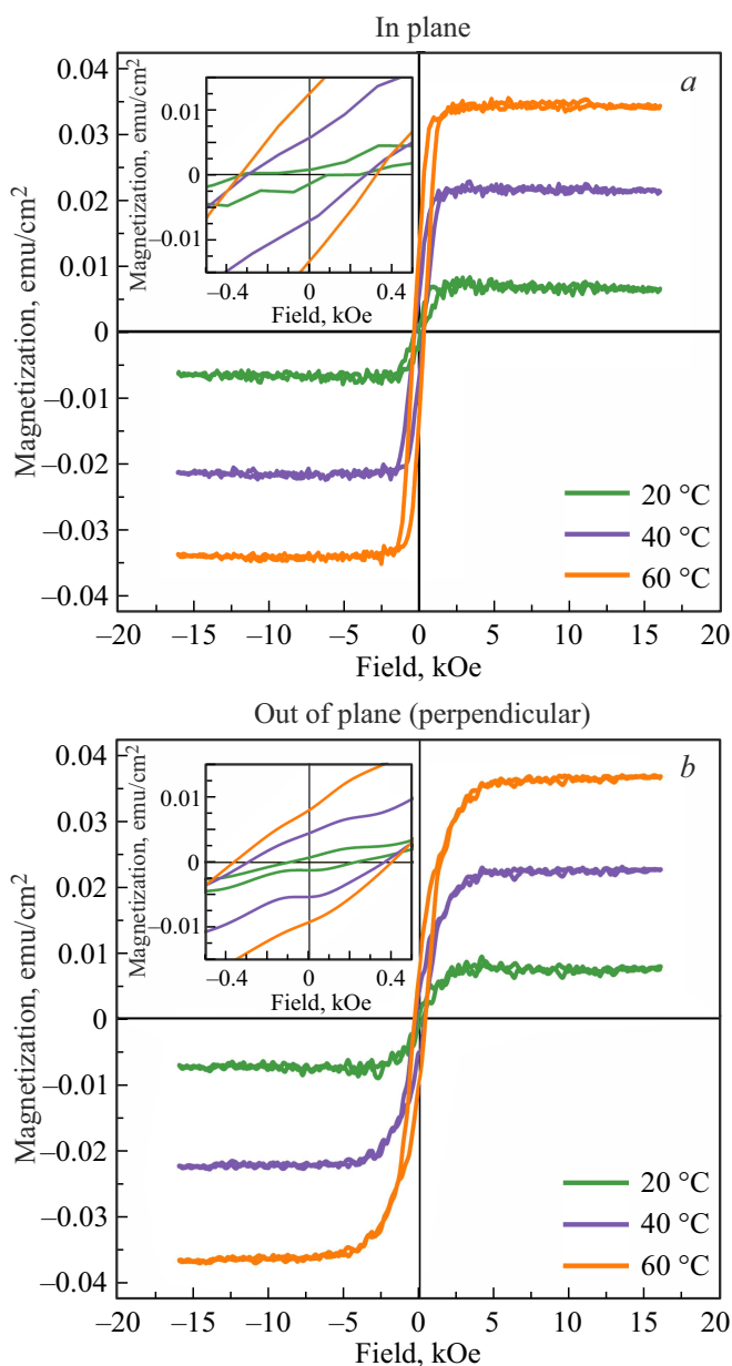
Рис. 4. Петли гистерезиса образцов Ni-НП, полученных при различных температурах (обозначены на рисунке), при различных ориентациях внешнего магнитного поля: а) in-plane, б) out-of-plane.
