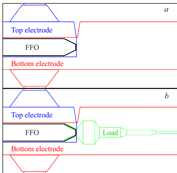
Рис. 3. Схематичное изображение неизлучающего конца РДП, вид сверху. a — РДП в традиционной геометрии; b — РДП с добавлением согласованной нагрузки. Top electrode, bottom electrode — верхний и нижний электроды соответственно (см. рис. 1). FFO — распределенный джозефсоновский переход. Load — согласованная нагрузка из молибдена.
