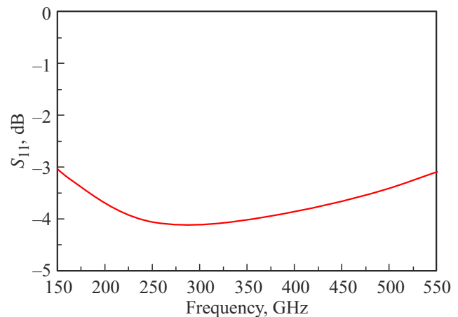
Рис. 5. Отношение амплитуды отраженной волны к амплитуде падающей волны, полученное для структуры, рассчитанной в Ansys HFSS.
