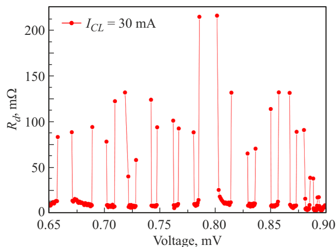
Рис. 2. Зависимость дифференциального сопротивления от напряжения для генератора без нагрузочных элементов при токе I_{CL} = 30 \text{ mA} . В явном виде наблюдаются области, в которых рабочие точки отсутствуют. При этих напряжениях для данного значения тока I_{CL} генерация невозможна.
