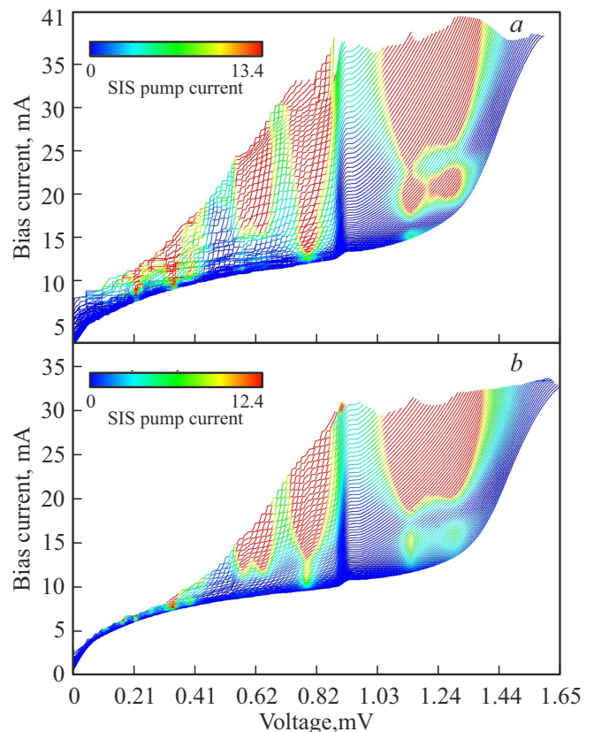
Рис. 7. Семейство вольтамперных характеристик РДП: a — без поглотителя, b — с поглотителем.
