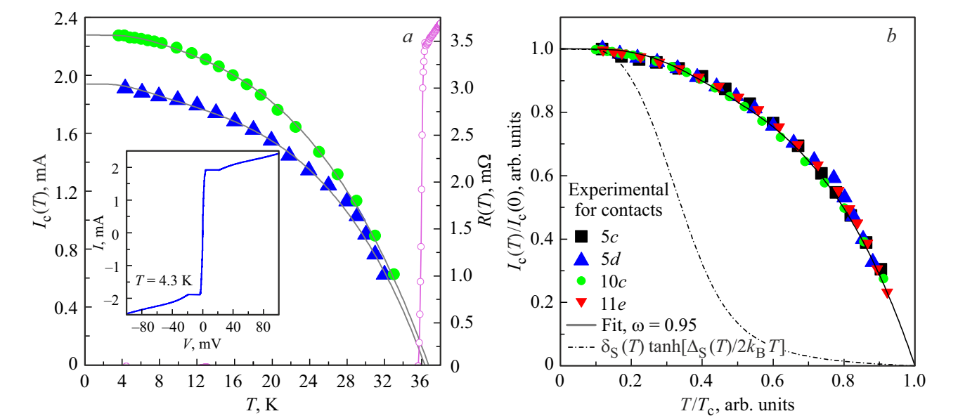
Рис. 7. a — температурные зависимости критического тока для двух СП-закоротов на базе CaKFe 4 As 4 (левая ось). Зависимость, построенная по данным рис. 6, приведена синими треугольниками; сплошные линии — упрощенная теоретическая аппроксимация I_c(T) . Светлые кружки — зависимость объемного сопротивления образца от температуры R(T) в районе перехода в СП-состояние (правая ось). На вставке показана ВАХ туннельного контакта с рис. 6 при T = 4.3 K в широком диапазоне напряжений смещения. b — зависимости критического тока от температуры в нормированных координатах. Помимо экспериментальных данных с панели „а“, красными треугольниками и черными квадратами приведены данные I_c(T)/I_c(0) для двух других контактов на базе поликристалла CaKFe 4 As 4 . Предельный случай \omega = 0 на основе аппроксимационной кривой \Delta_S(T) (рис. 3, b ) показан пунктирной линией, аппроксимация формулой (2) показана сплошной линией.
