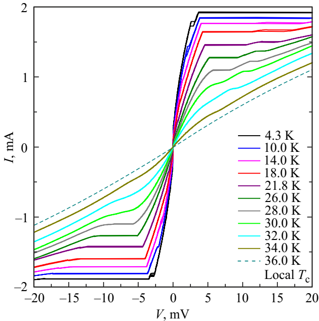
Рис. 6. ВАХ сверхпроводящей закоротки, подключенной последовательно с SnS-андреевским контактом на базе поликристалла \text{CaKFe}_4\text{As}_4 . Измерено в диапазоне T = 4.2\text{--}36.0\text{ K} . Токовые плато на ВАХ соответствуют критическим токам перехода СП-закоротки в нормальное состояние с конечным сопротивлением. Штриховой линией показана ВАХ этого туннельного контакта в нормальном состоянии при локальной T_c = 36.0\text{ K} .
