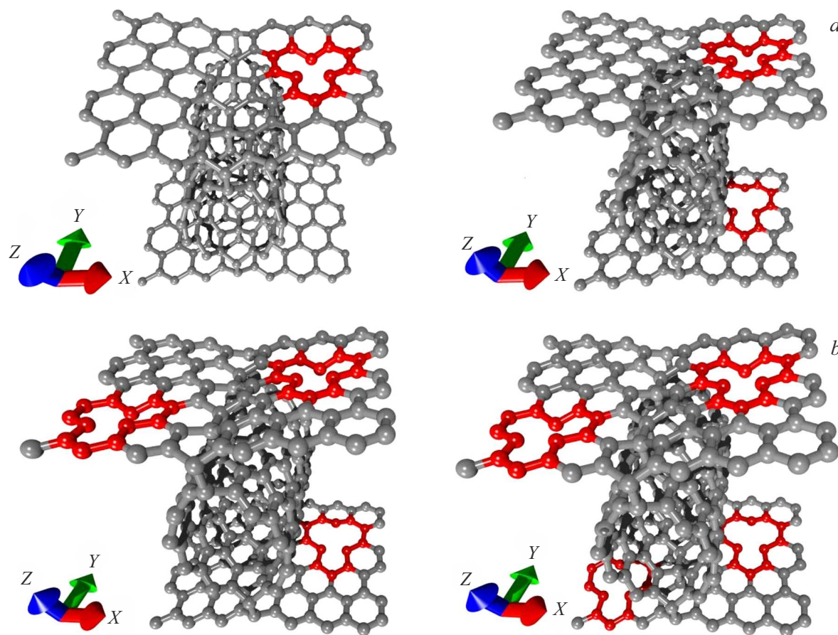
Рис. 2. Супер-ячейка гибридной пленки графен-ОУНТТ (10,0)-графен с дефектами типа одиночная вакансия, формируемыми в атомной сетке листов графена: один (a), два (b), три (c) и четыре (d) дефекта. Красным цветом выделены области локализации дефекта.
