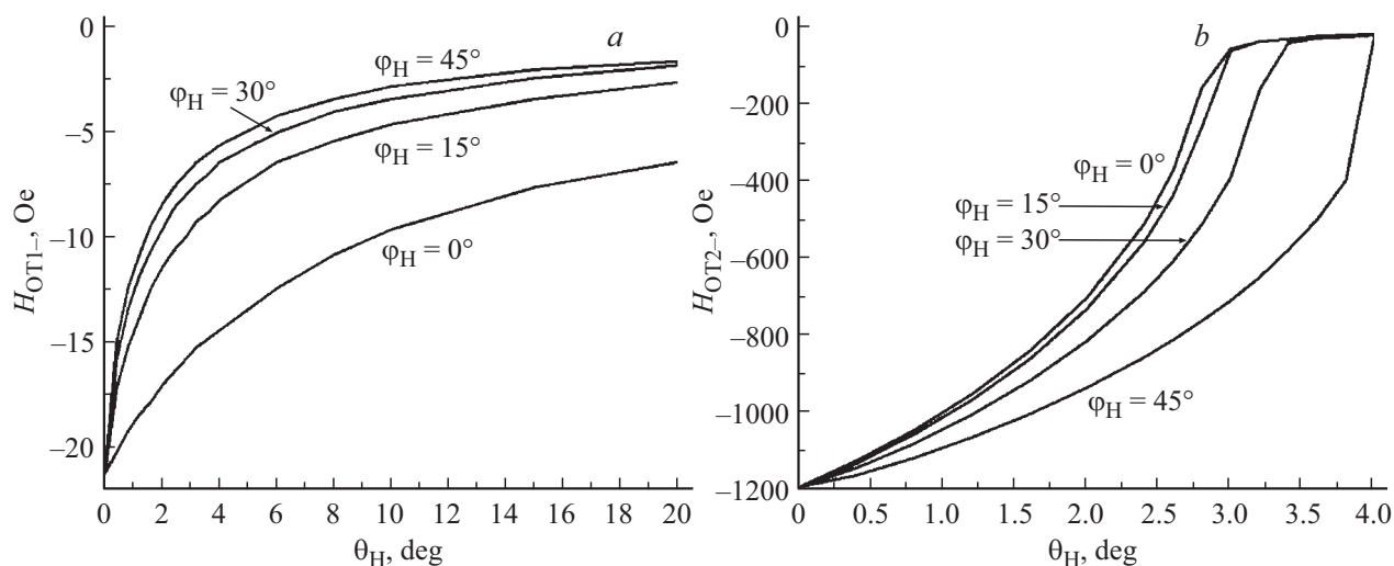
Рис. 7. Угловые зависимости от \theta_H полей ОП1- (a) и ОП2- (b) для \varphi_H = 0^\circ, 15^\circ, 30^\circ и 45^\circ .
