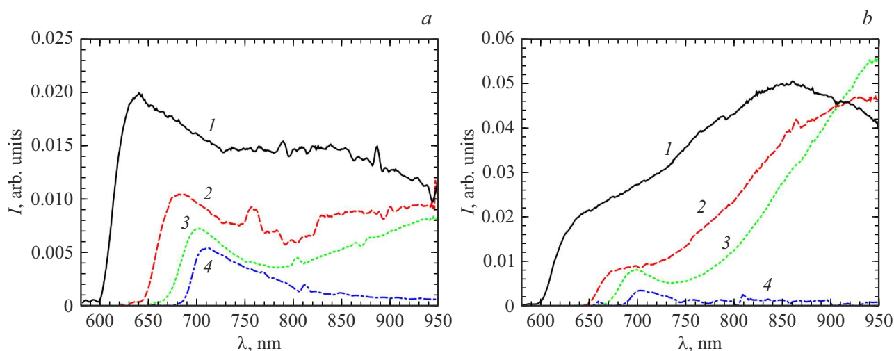
Рис. 1. (а) Спектры люминесценции красных цветных стекол КС в полосе их пропускания при возбуждении лазерным излучением на длинах волн 405 (а) и 510 nm (b). Обозначения фильтров на рис. а и b: 1 — KC11, 2 — KC17, 3 — KC18, 4 — KC19.
