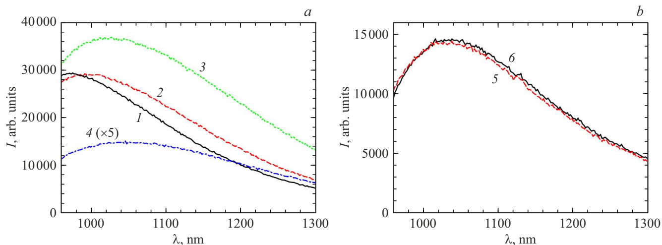
Рис. 2. (а) Спектры ИК люминесценции фильтров типа КС при возбуждении на длине волны 405 nm: KC11 (1), KC17 (2), KC18 (3), KC19 (4). Для фильтра KC19 на графике представлен сигнал люминесценции, увеличенный в 5 раз по отношению к реальному. (b) Спектры ИК люминесценции фильтров ИКС3 (5) и ИКС7 (6) при возбуждении на длине волны 405 nm.
