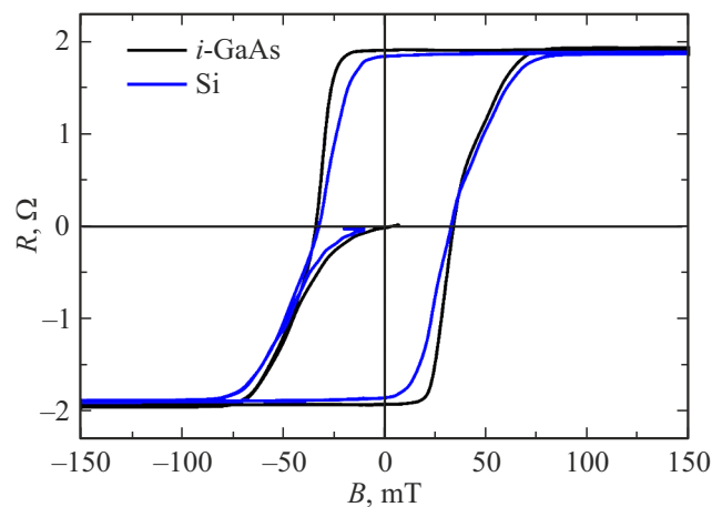
Рис. 2. Экспериментально полученные магнитолевые зависимости сопротивления Холла при 300 K пленок, сформированных на подложках полуизолирующего арсенида галлия ( i -GaAs, черная кривая) и кремния (Si, синяя кривая).
