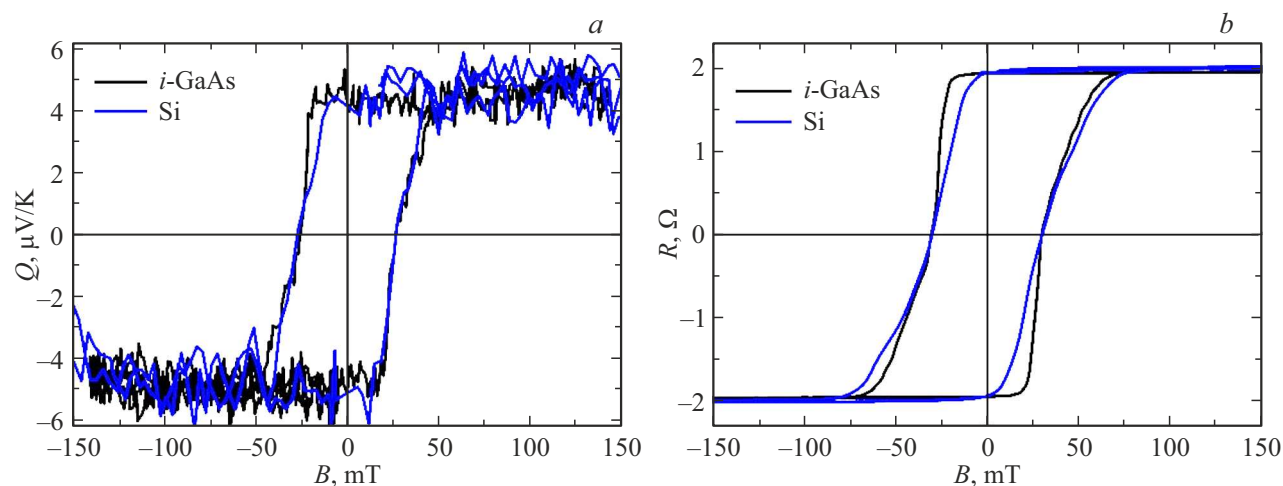
Рис. 4. Сопоставление экспериментально полученных магнито-транспортных зависимостей коэффициентов Нернста–Эттингсгаузена (а) и сопротивлений Холла (b) исследуемых образцов при средней температуре 345 К.
