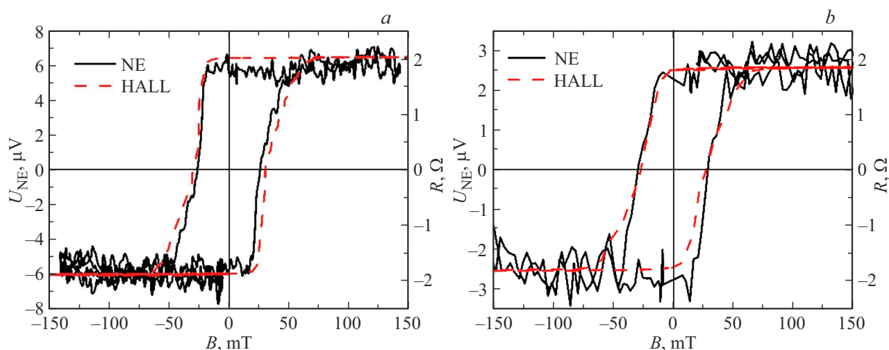
Рис. 3. Сопоставление экспериментально полученных магнито-транспортных зависимостей сопротивления Холла и напряжения Нернста–Эттингсгаузена пленки, сформированной на подложках i -GaAs (а) и Si (b).
