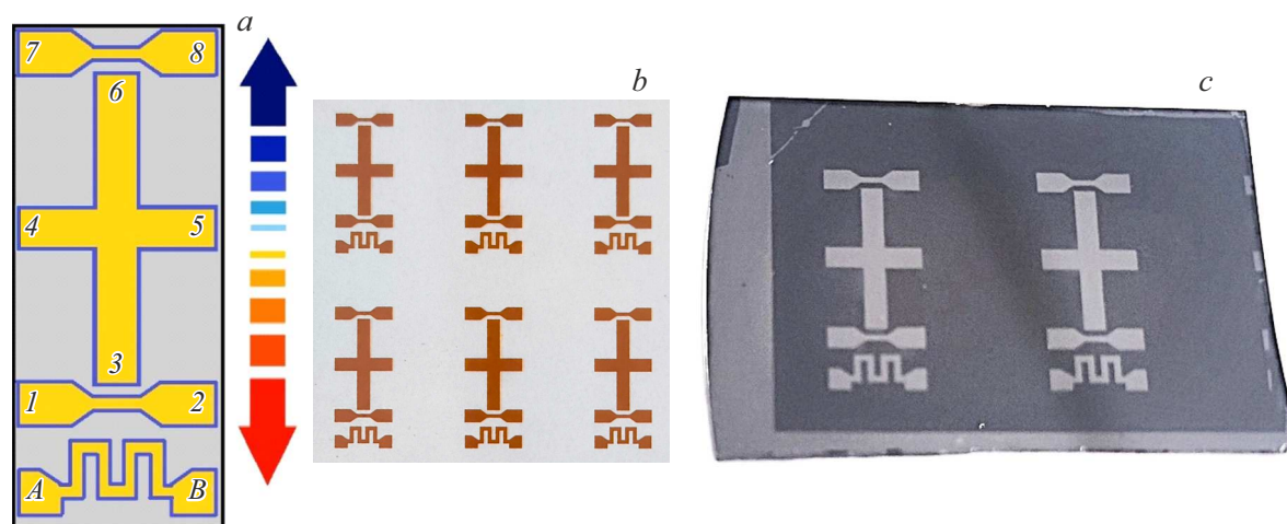
Рис. 1. a — топология пленки для измерений гальваномагнитных, термоэлектрических и термомагнитных эффектов: 1–2, 7–8 — терморезисторы, 3–4–5–6 — контакты для измерений эффектов Холла и Нернста–Эттингсгаузена, А–В — резистор-нагреватель; b — фотошаблон; c — фотография образца с литографическим рисунком.
