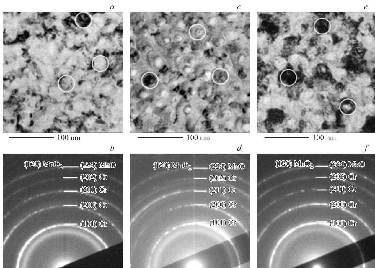
Рис. 4. ПЭМ-фотографии ( a, c, e ) и электронограммы ( b, d, f ) пленок Ta/Cr 70 Mn 30 ( L )/Ta с L = 20 nm ( a, b ) и L = 50 nm ( e, f ), а также пленки Ta/Cr 70 Mn 30 (20)/Fe 20 Ni 80 /Ta ( c, d ). Белыми окружностями обозначены типичные элементы структуры, являющиеся отдельными кристаллами.
