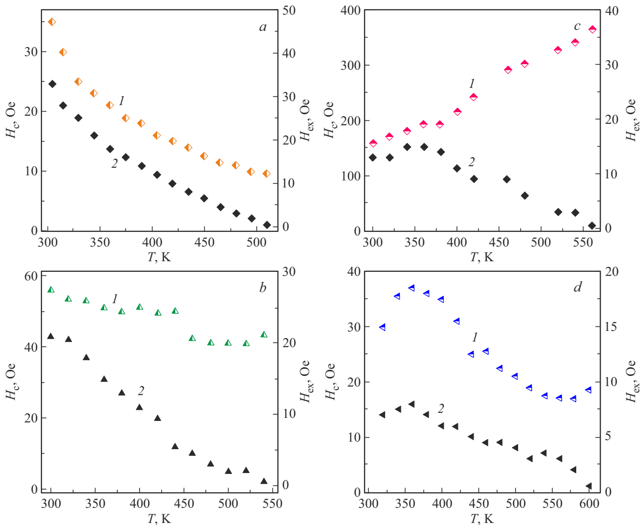
Рис. 2. Температурные зависимости коэрцитивной силы H_c (кривые 1) и поля обменного смещения H_{ex} (кривые 2) для пленок с различными ферромагнитными слоями: a — \text{Fe}_{20}\text{Ni}_{80} ( L = 50 nm); b — \text{Fe} ( L = 100 nm); c — \text{Fe}_{10}\text{Co}_{90} ( L = 300 nm); d — \text{Fe}_{60}\text{Co}_{20}\text{B}_{20} ( L = 210 nm).
