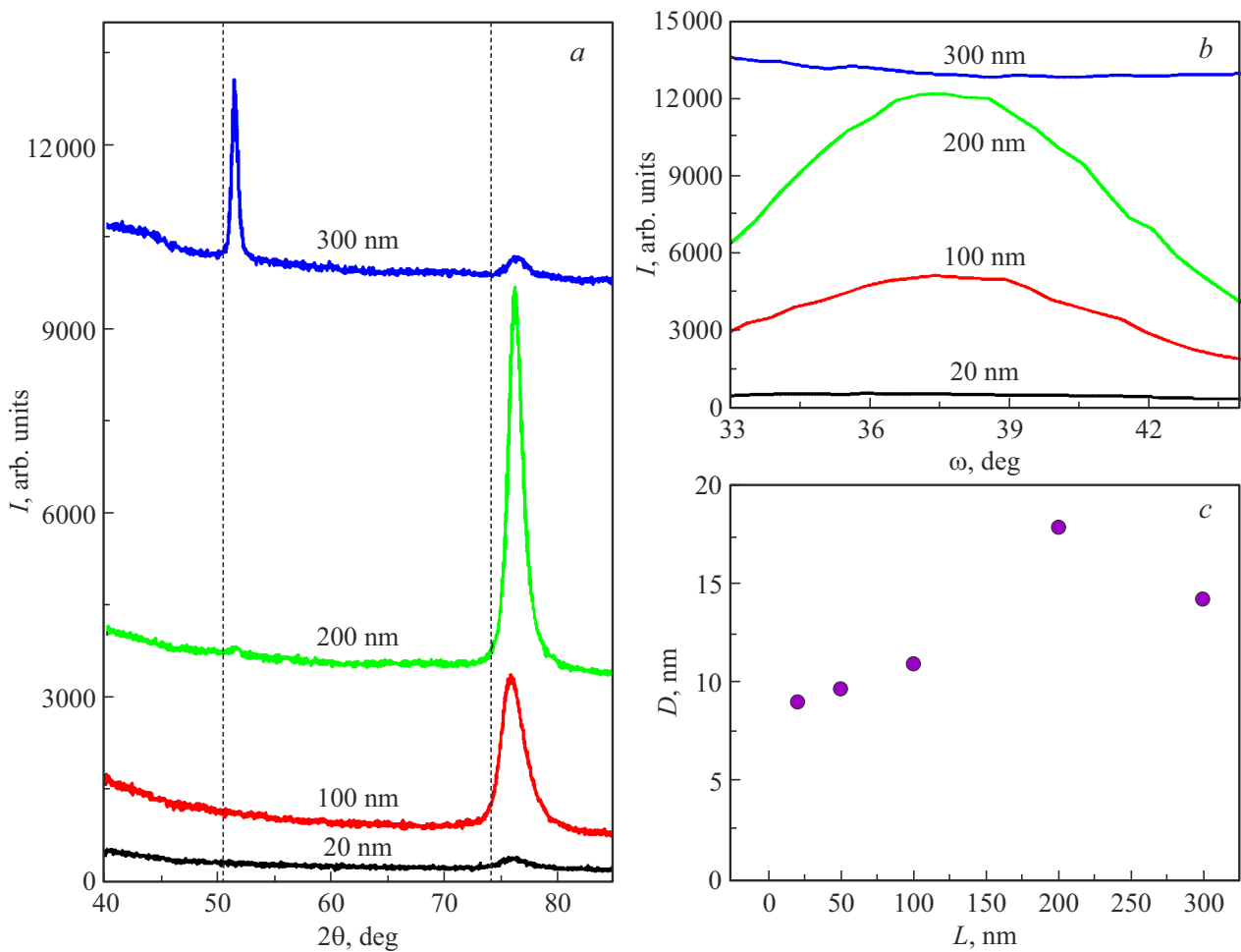
Рис. 3. a — Дифрактограммы пленок Ta/Cr 70 Mn 30 ( L )/Ta с различной толщиной L слоя Cr–Mn. b — Кривые качания дифракционных линий вблизи угла дифракции 2\theta = 75.50^\circ . c — Зависимость среднего диаметра кристаллитов, определенного по формуле Шерера, от толщины слоя Cr–Mn.
