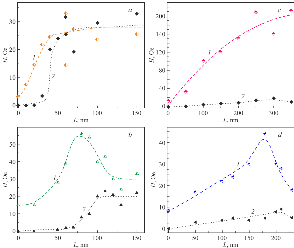
Рис. 1. Зависимости коэрцитивной силы H_c (кривые 1) и поля обменного смещения H_{ex} (кривые 2) от толщины L слоя Cr–Mn для пленок с различным ферромагнитными слоями: Fe_{20}Ni_{80} (a), Fe (b), Fe_{10}Co_{90} (c), Fe_{60}Co_{20}B_{20} (d).
