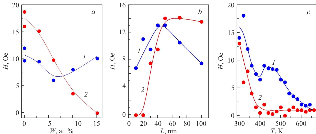
Рис. 5. Зависимости коэрцитивной силы (кривая 1) и поля обменного смещения (кривая 2) от концентрации W в пленках (Cr_{70}Mn_{30})_{100-x}W_x(50 nm)/Fe_{20}Ni_{80} (a), от толщины антиферромагнитного слоя в пленках (Cr_{70}Mn_{30})_{95}W_5(L)/Fe_{20}Ni_{80} (b), полученные при температуре 300 K, и от температуры в пленках (Cr_{70}Mn_{30})_{95}W_5(50 m)/Fe_{20}Ni_{80} (c).
