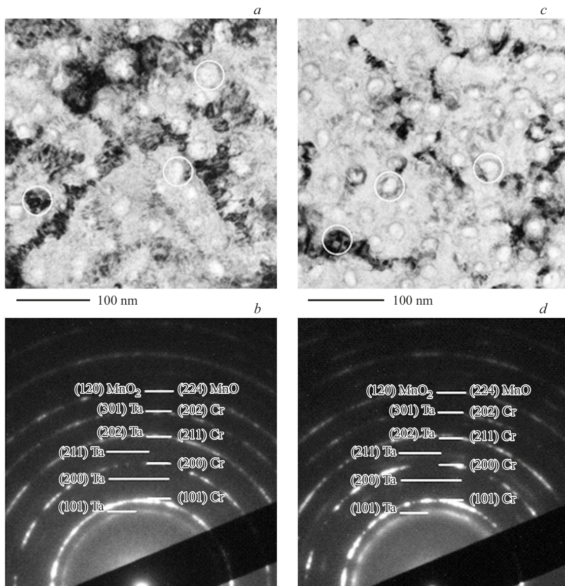
Рис. 6. ПЭМ-фотографии ( a, c ) и электронограммы ( b, d ) пленок Ta/(Cr 70 Mn 30 ) 95 W 5 (L)/Ta с L = 20 nm ( a, b ) и L = 50 nm ( c, d ). Белыми окружностями обозначены типичные элементы структуры, являющиеся отдельными кристаллами.
