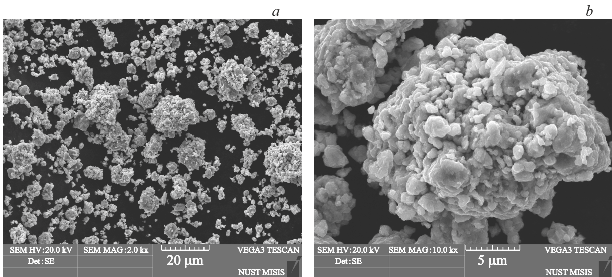
Рис. 2. Микрофотографии (СЭМ) порошка после измельчения.
