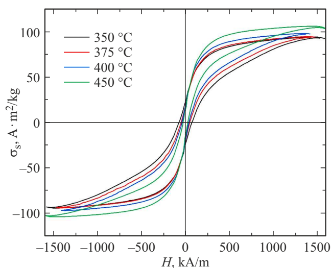
Рис. 3. Петли магнитного гистерезиса образцов после отжига.
