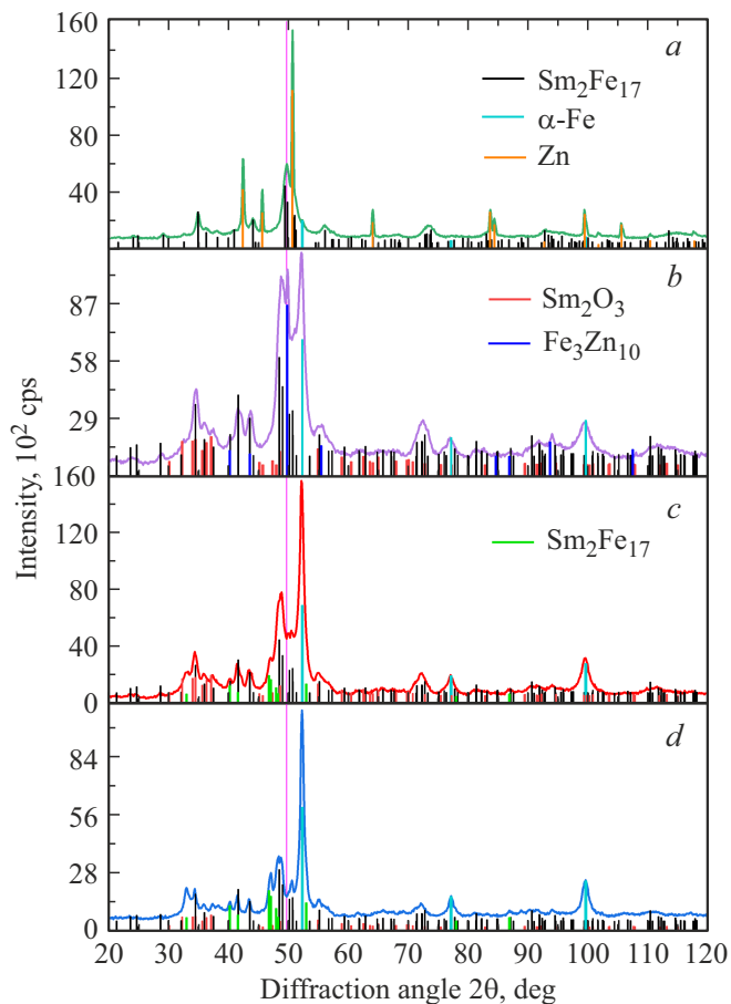
Рис. 1. Рентгеновские спектры образцов: а) после измельчения с добавлением Zn; после последующего отжига при: б) 350 °C, в) 400 °C, д) 450 °C.
