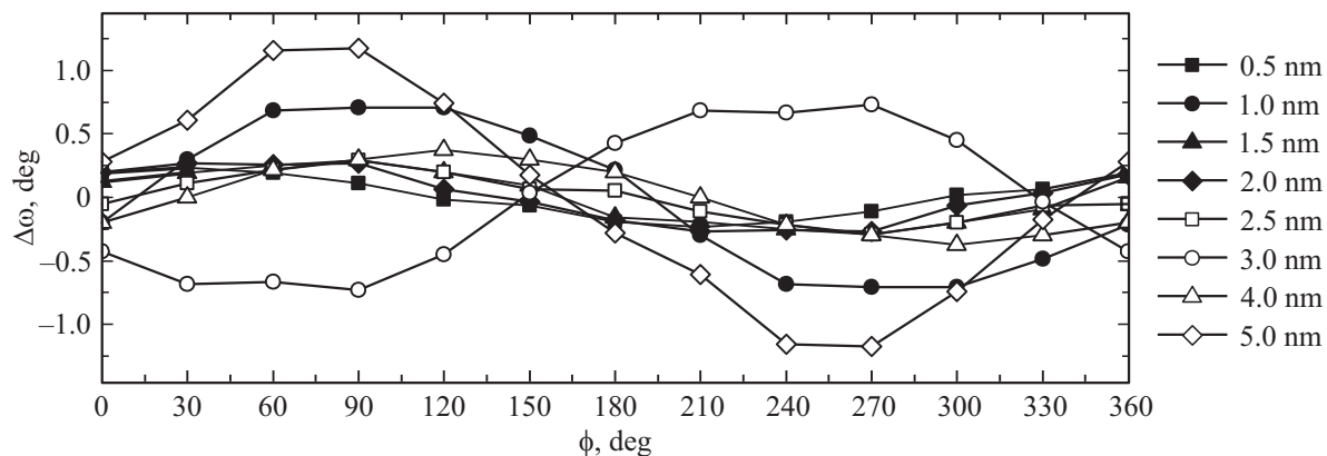
Рис. 4. Зависимость невязимности \Delta\omega структур от угла поворота для разных значений толщины слоя Nb d_2 .
