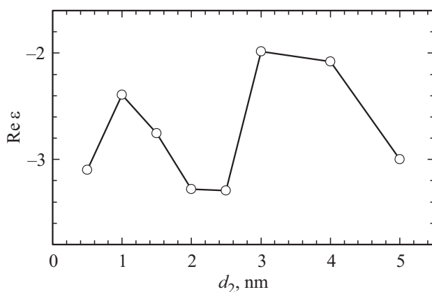
Рис. 2. Зависимость эффективной диэлектрической проницаемости исследованных структур от толщины слоя Nb d_2 .
