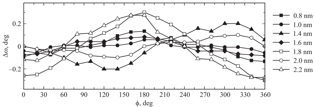
Рис. 5. Зависимость невязности \Delta\omega структур от угла поворота для разных значений толщины слоев FeNi.
