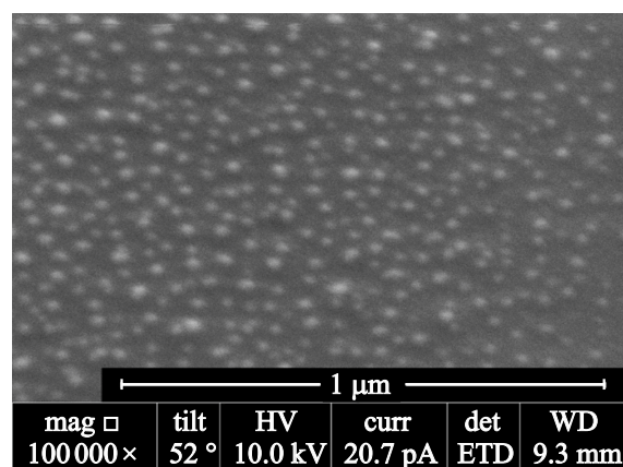
Рис. 1. Типичный вид островковой пленки FeNi на ситаловой подложке [10].
