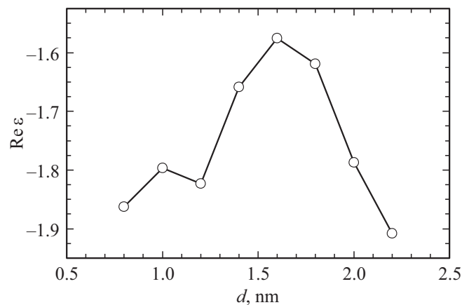
Рис. 3. Зависимость эффективной диэлектрической проницаемости исследованных структур от толщины слоев FeNi.
