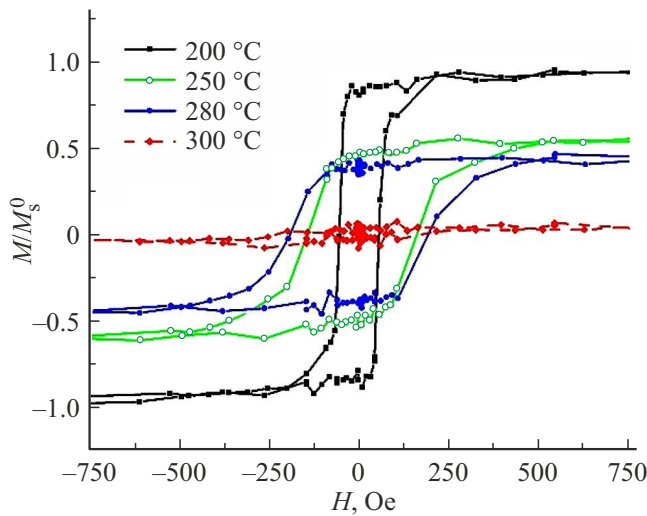
Рис. 6. Петли магнитного гистерезиса \text{MgO}(100)/^{57}\text{Fe}(50 \text{ nm})/\text{Cr}(2 \text{ nm}) после отжига при температурах 200, 250, 280, 300 °C. Длительность отжига — 60 min.
