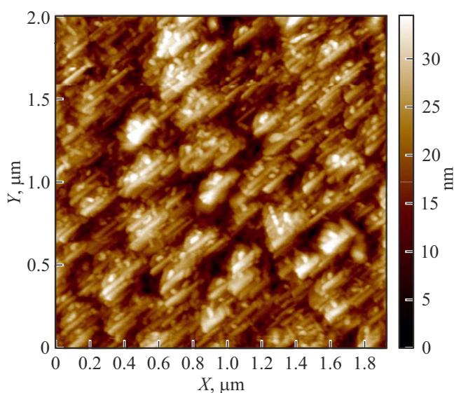
Рис. 10. АСМ-изображение поверхности образца \text{MgO}/^{57}\text{Fe}(50 \text{ nm})/\text{Cr}(2 \text{ nm}) после T_a = 250^\circ\text{C} .
