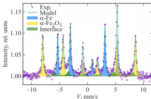
Рис. 9. Мёсбауэровский спектр (CEMS) \text{MgO}/^{57}\text{Fe}(50\text{ nm})/\text{Cr}(2\text{ nm}) после отжига при T_a = 250^\circ\text{C} ( t = 60\text{ min} ).
