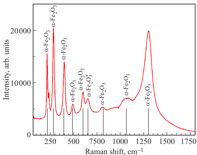
Рис. 8. Спектр комбинационного рассеяния света \text{MgO}/\text{Fe}(50\text{ nm})/\text{Cr}(2\text{ nm}) после отжига при T_a = 250^\circ\text{C} .
