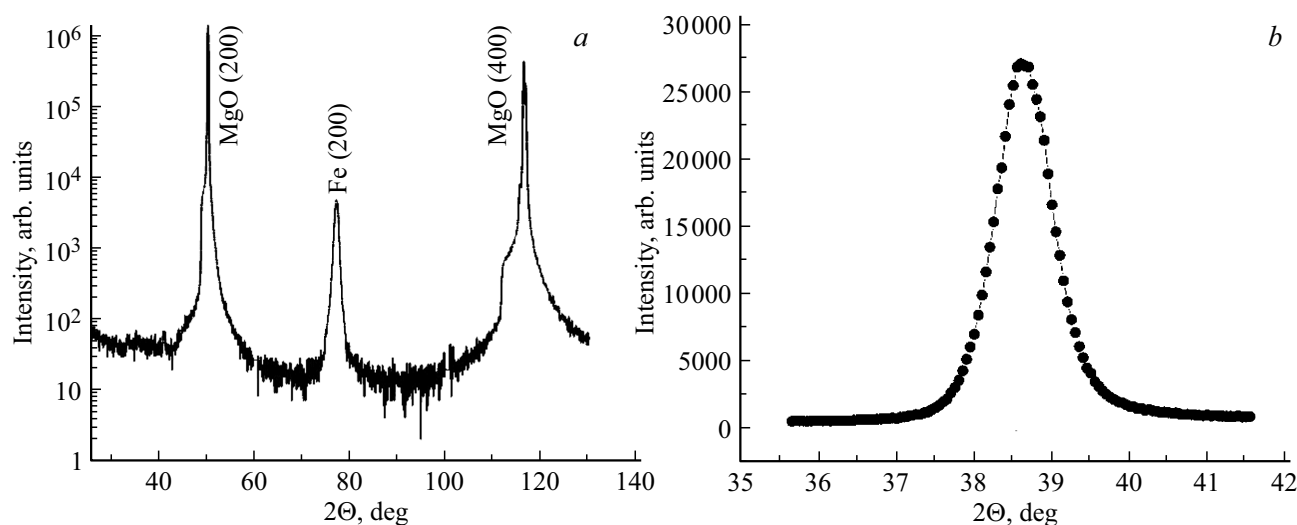
Рис. 1. a — Рентгеновская дифрактограмма образца \text{MgO}/^{57}\text{Fe}(50\text{ nm})/\text{Cr}(2\text{ nm}) ; b — кривая качания, измеренная на дифракционной линии (200) Fe.
