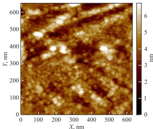
Рис. 3. АСМ-изображение поверхности образца \text{MgO}/\text{Fe}(50\text{ nm})/\text{Cr}(2\text{ nm}) .
