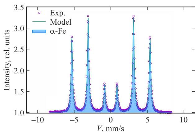
Рис. 4. Мёссбауэровский спектр (CEMS) пленки \text{MgO}(100)/^{57}\text{Fe}(50 \text{ nm})/\text{Cr}(2 \text{ nm}) .
