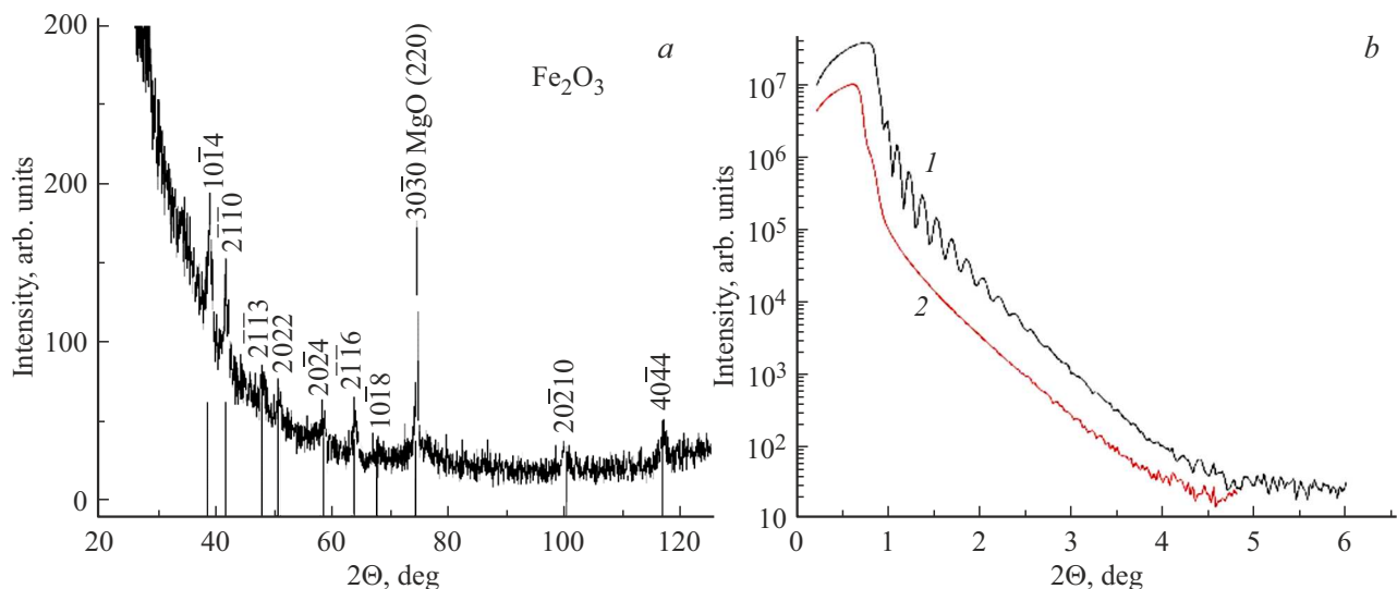
Рис. 7. а — GIXRD дифрактограмма образца \text{MgO}/^{57}\text{Fe}(50 \text{ nm})/\text{Cr}(2 \text{ nm}) после отжига при T_a = 250 °C-60 min; б — кривые отражения рентгеновской рефлектометрии образца \text{MgO}/^{57}\text{Fe}(50 \text{ nm})/\text{Cr}(2 \text{ nm}) до (1) и после (2) отжига T_a = 250 °C ( t = 60 min).
