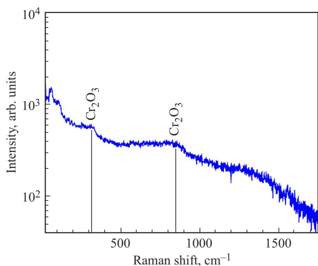
Рис. 2. Спектр комбинационного рассеяния света \text{MgO}/^{57}\text{Fe}(50\text{ nm})/\text{Cr}(2\text{ nm}) .
