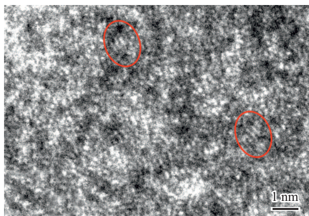
Рис. 4. Электронно-микроскопическое изображение структуры ленты 2HCP после термомагнитной обработки при 540 °C в течение 7 min. Выделены области с квазиупорядоченным расположением рассеивающих центров.
