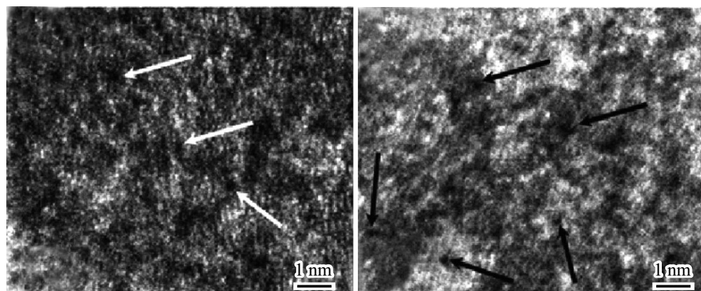
Рис. 3. Электронно-микроскопические изображения структуры ленты 2НСП после термомагнитной обработки при 540°С в течение 7 min. Стрелками указаны частицы (предположительно) второй фазы.
