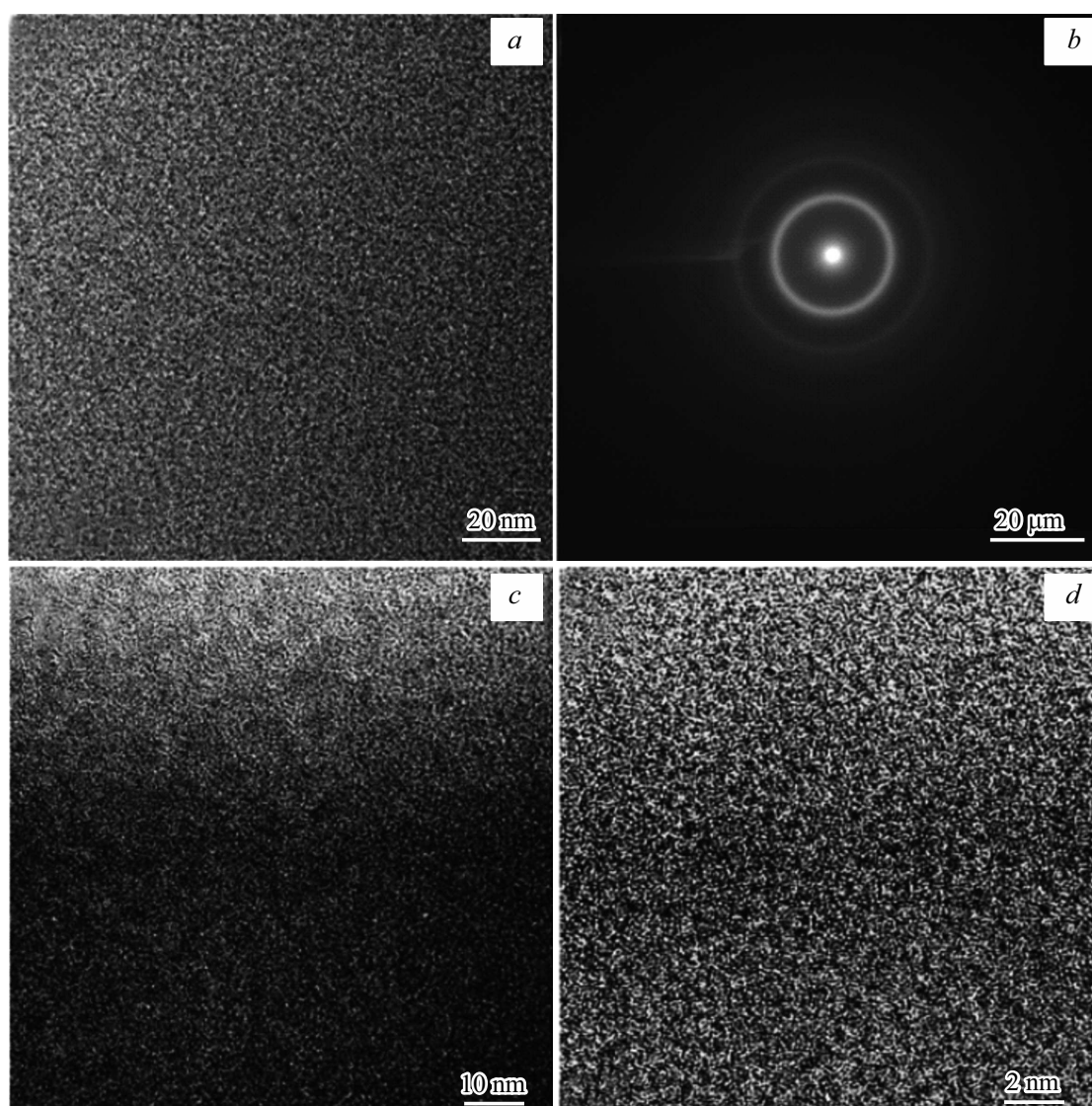
Рис. 2. Электронно-микроскопическое изображение структуры ленты 2НСП после термомагнитной обработки при 540°С в течение 7 min. a, c, d — светопольные изображения, полученные при различном увеличении; b — микроэлектроннограмма участка, представленного на части a .
