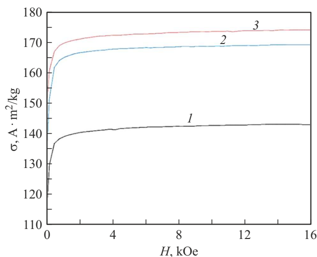
Рис. 1. Изменение намагниченности насыщения в зависимости от величины внешнего магнитного поля для образцов сплава 2НСП. 1 — исходное состояние; 2, 3 — ТУО в течение 5 и 7 min соответственно.
