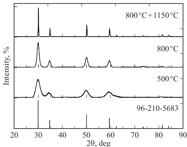
Рис. 1. Дифрактограммы твердых растворов ZrO_2 - 30 \text{ mol.}\% Yb_2O_3 , подвергнутых отжигу при различных температурах. PDF-96-210-5683 — кубическая фаза [11].
