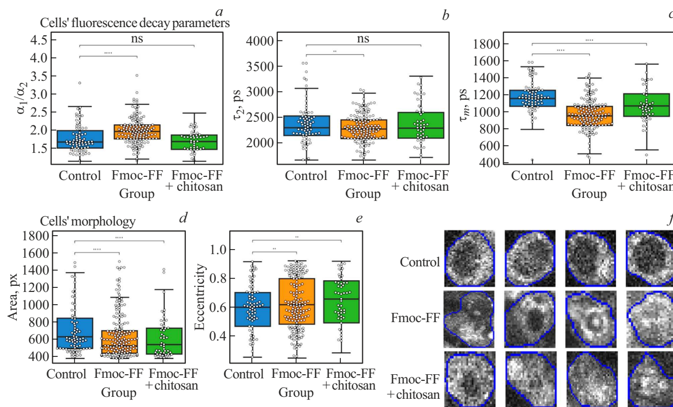
Рис. 4. Распределение параметров (a) отношения амплитуд быстрой и медленной компонент \alpha_1/\alpha_2 , (b) времени затухания \tau_2 , (c) среднего времени \tau_m , (d) площади и (e) эксцентриситета маски сегментации для клеток MCF-7 на чашке Петри (контроль) (синие столбцы), на гидрогеле Fmoc-FF (оранжевые столбцы) и MCF-7 на гидрогеле Fmoc-FF+хитозан (зеленые столбцы). (f) Характерные примеры сегментированных клеток групп контроля, Fmoc-FF и „Fmoc-FF+хитозан“.
