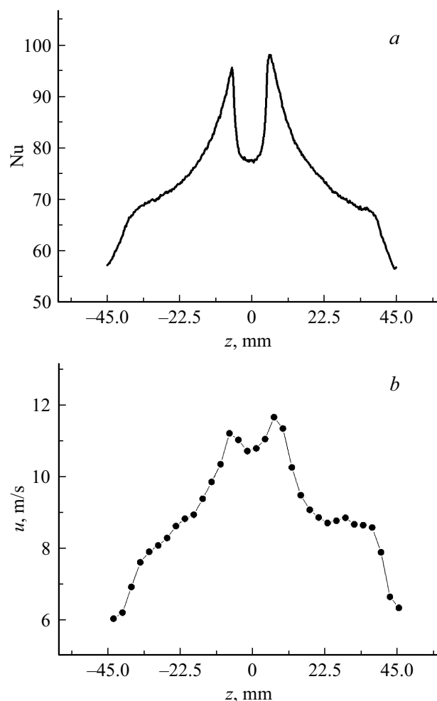
Рис. 2. Распределение коэффициента теплоотдачи (а) и распределение скорости на расстоянии 5h от стенки (б). Координата z отсчитывается от оси симметрии стенки.
