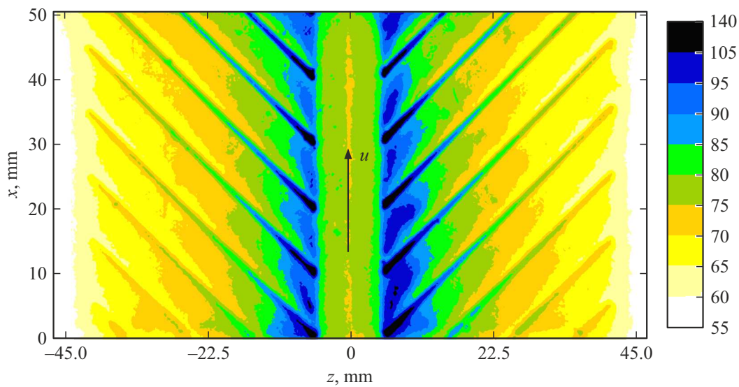
Рис. 1. Распределение коэффициента теплоотдачи на стенке. Направление потока указано стрелкой.
