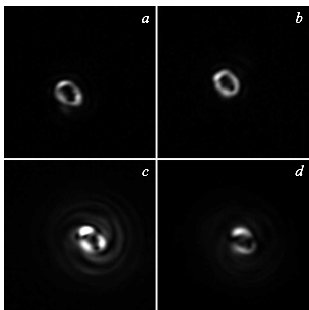
Рис. 4. Профили отражённого от WG1 (a) и WG2 (b) пучка в ближнем поле на длине волны резонанса; c, d — то же с наложением референсного пучка.
