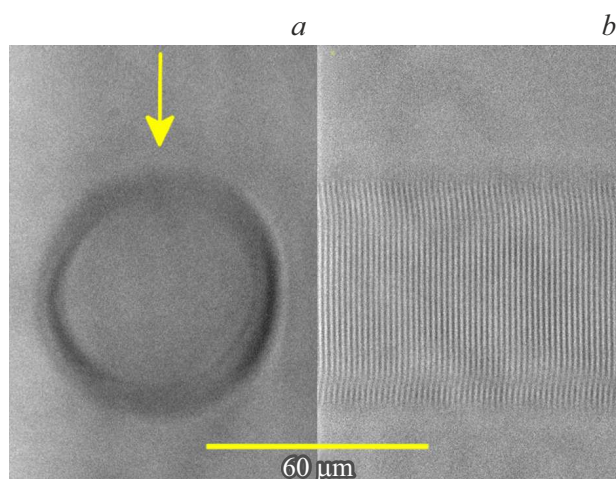
Рис. 1. (a) Микроснимок WG1 с торца. Направление пучка фемтосекундного лазера обозначено стрелкой; (b) вид WG1 вдоль направления записывающего пучка. Масштабная линия относится к обоим видам, подсветка снизу.
