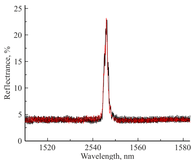
Рис. 3. Спектры отражения волноводов. WG1 — чёрная сплошная линия, WG2 — красная пунктирная линия.
