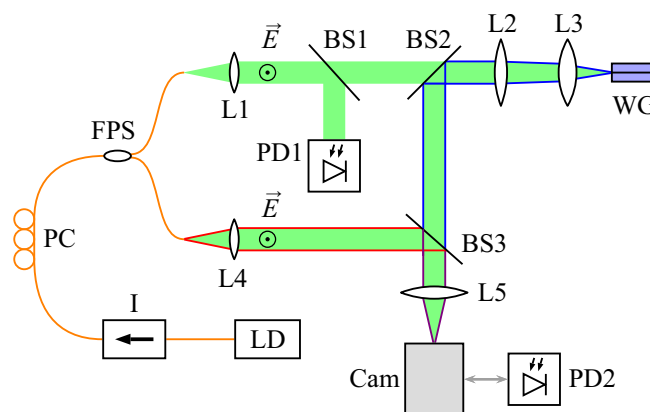
Рис. 2. Оптическая схема для характеристики волноводов. LD — полупроводниковый лазер с изменяемой длиной волны; I — волоконно-оптический изолятор; PC — контроллер поляризации; FPS — волоконно-оптический делитель; L1, 2, 3, 4, 5 — линзы с фокусными расстояниями 10, 500, 50, 20, 400 mm соответственно; BS1, 2, 3 — делители пучка; Cam — InGaAs-камера; PD1, 2 — фотодиоды; WG — образец фосфатного стекла с исследуемыми волноводами.
