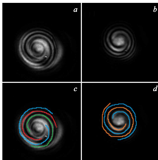
Рис. 5. Профили отражённого от WG1 (a) и WG2 (b) пучка в дальнем поле. То же с наложением схемы рукавов спирали: 3 рукава для WG1 (c), 2 рукава для WG2 (d).
