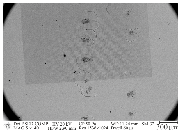
Рис. 1. Фотография образца 1 в окрестности микроструктуры АМП 1.1 после воздействия.
