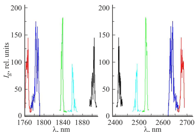
Рис. 5. Полученные спектры перестраиваемого выходного двухмикронного излучения: красные линии — пара 1766 и 2677 nm; синие линии — 1784 и 2636 nm; зеленые линии — 1838 и 2527 nm; голубые линии — 1858 и 2490 nm; черные линии — 1900 и 2418 nm.
