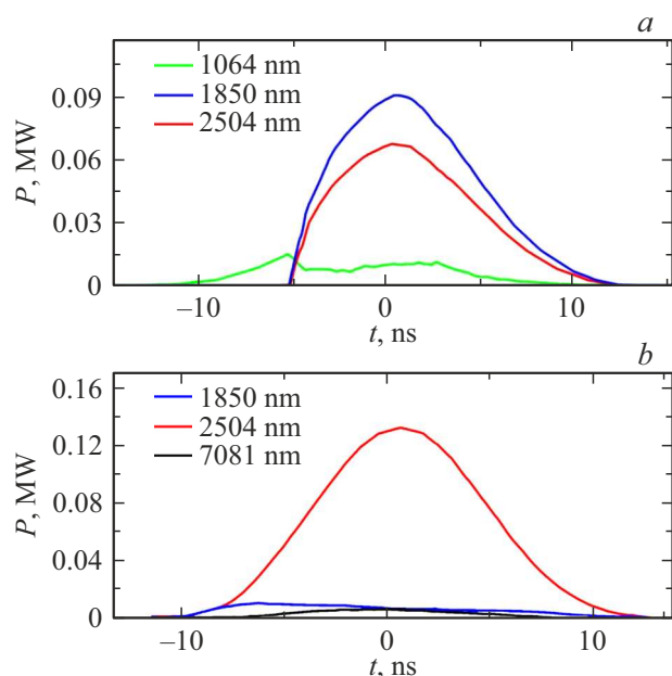
Рис. 4. Результаты моделирования двухкаскадного ПГС: (a) преобразование в KTP на первом этапе расчета; (b) преобразование в LGSe на втором этапе расчета.
