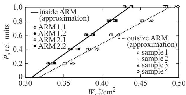
Рис. 2. Зависимости вероятности пробоя от плотности энергии излучения: ARM 1.1 (или АМП 1.1) — первая микроструктура образца 1; ARM 1.2 (или АМП 1.2) — вторая микроструктура образца 1; ARM 2.1 (или АМП 2.1) — первая микроструктура образца 2; ARM 2.2 (или АМП 2.2) — вторая микроструктура образца 2; sample 1 и sample 2 — образцы 1 и 2 вне микроструктур; sample 3 и sample 4 — образцы 3 и 4 без микроструктур.
