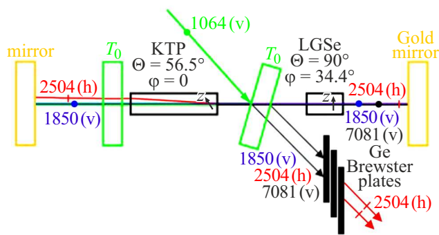
Рис. 3. Оптическая схема двухкаскадного ПГС на кристаллах KTP и LGSe: кристаллооптические оси Z кристаллов KTP и LGSe ориентированы в горизонтальной плоскости (плоскость рисунка); (v) — вертикальная поляризация излучения; (h) — горизонтальная поляризация излучения.
