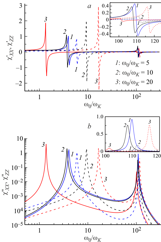
Рис. 6. Действительная \chi'_{GG} (a) и мнимая \chi''_{GG} (b) части компоненты тензора линейной восприимчивости \chi_{GG} = \chi'_{GG} - i\chi''_{GG} (уравнение (33)) АФМ в зависимости от \omega/\omega_K для \alpha = 0.01 , \tau\omega_K = 0.001 , \omega_\Lambda/\omega_K = 10 и различных значений \omega_0/\omega_K , соответствующих состоянию (d). Сплошные линии: G = X , штриховые линии: G = Z .
