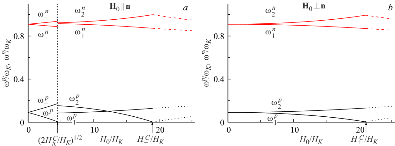
Рис. 3. Мнимые части \omega_i^{p,n} = \text{Im}[\omega_i^{p,n}] комплексных частот прецессии и нутации намагниченности АФМ в зависимости от величины внешнего поля H_0 для \alpha = 0.01 , \tau\omega_K = 0.01 , \omega_\Lambda/\omega_K = 10 : (а) поле направлено вдоль легкой оси; (б) поле направлено перпендикулярно легкой оси.
