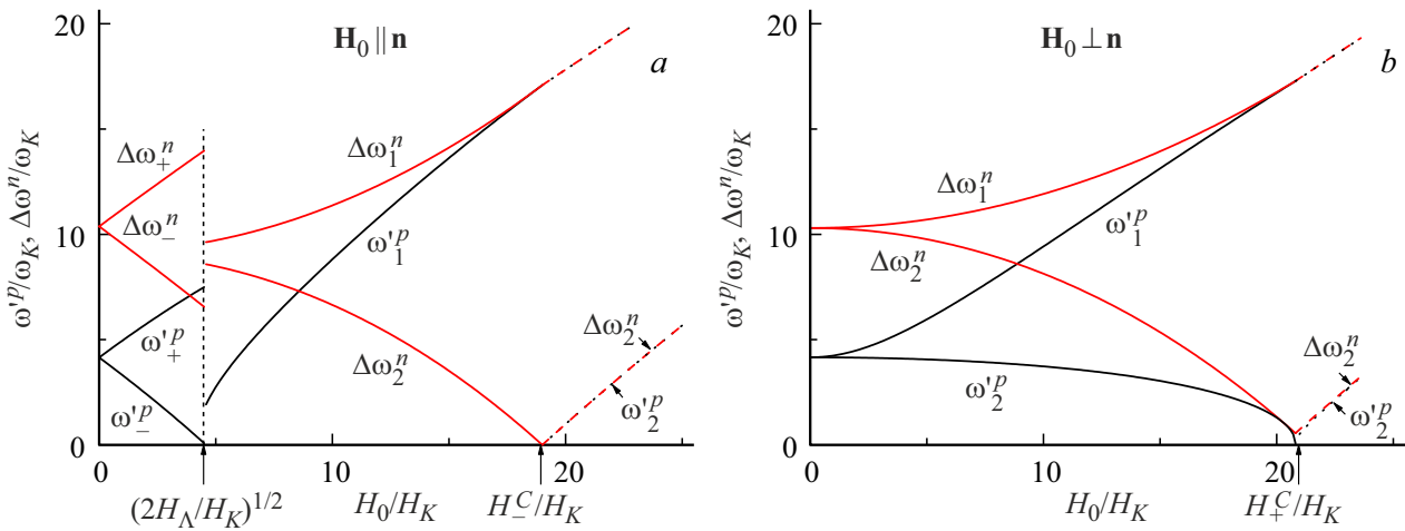
Рис. 2. Частота прецессии \omega_i^p = \text{Re}[\omega_i^p] суммарной намагниченности подрешеток АФМ и отклонение нутационной частоты намагниченности \Delta\omega_i^n = \text{Re}[\omega_i^n] - 1/\tau в зависимости от величины внешнего поля H_0 для \alpha = 0.01 , \tau\omega_K = 0.01 , \omega_\Lambda/\omega_K = 10 : (а) поле направлено вдоль легкой оси; (б) поле направлено перпендикулярно легкой оси.
