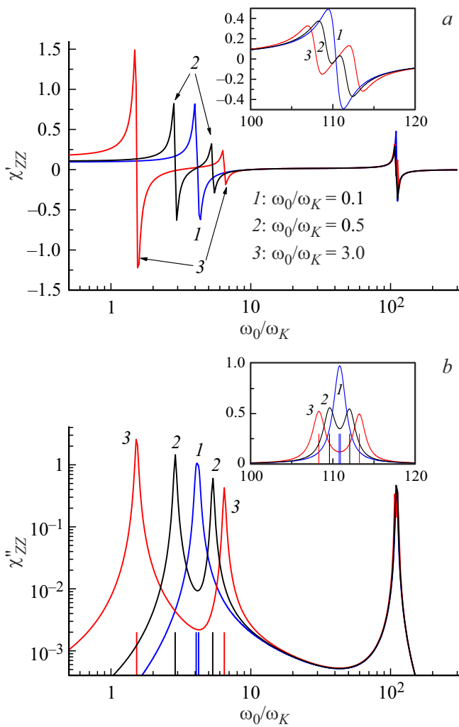
Рис. 4. Действительная \chi'_{zz} (a) и мнимая \chi''_{zz} (b) части компоненты тензора линейной восприимчивости \chi_{zz} = \chi'_{zz} - i\chi''_{zz} (уравнение (33)) АФМ в зависимости от \omega/\omega_K для \alpha = 0.01 , \tau\omega_K = 0.001 , \omega_\Lambda/\omega_K = 10 и различных значений \omega_0/\omega_K , соответствующих состоянию (a). Частотные метки — решения уравнения (a) из табл. 2 для \alpha = 0 .
