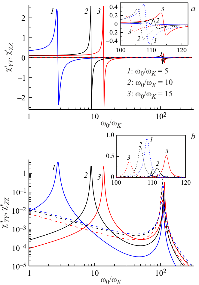
Рис. 5. Действительная \chi'_{GG} (a) и мнимая \chi''_{GG} (b) части компоненты тензора линейной восприимчивости \chi_{GG} = \chi'_{GG} - i\chi''_{GG} (уравнение (33)) АФМ в зависимости от \omega/\omega_K для \alpha = 0.01 , \tau\omega_K = 0.001 , \omega_\Lambda/\omega_K = 10 и различных значений \omega_0/\omega_K , соответствующих состоянию (b). Сплошные линии: G = Z , штриховые линии: G = Y .
