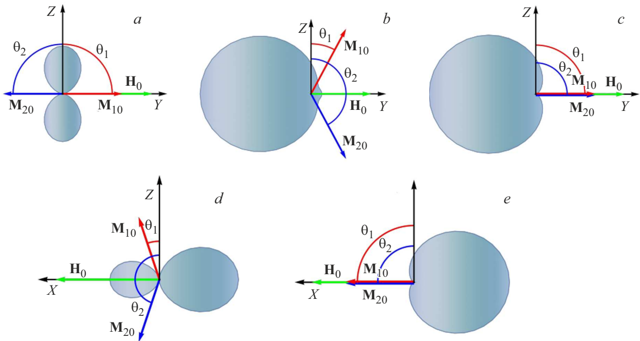
Рис. 1. Геометрия задачи: a–c — легкая ось расположена вдоль оси Y , \mathbf{n} = \mathbf{e}_Y , внешнее поле направлено вдоль легкой оси \mathbf{H}_0 = H_0 \mathbf{e}_Y ; d, e — легкая ось расположена вдоль оси Z , \mathbf{n} = \mathbf{e}_Z , внешнее магнитное поле \mathbf{H}_0 приложено перпендикулярно легкой оси \mathbf{H}_0 = H_0 \mathbf{e}_X .
