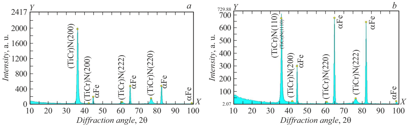
Рис. 6. Дифрактограммы покрытий состава Ti–Cr–N. a — 5; b — 17 at.% хрома.
