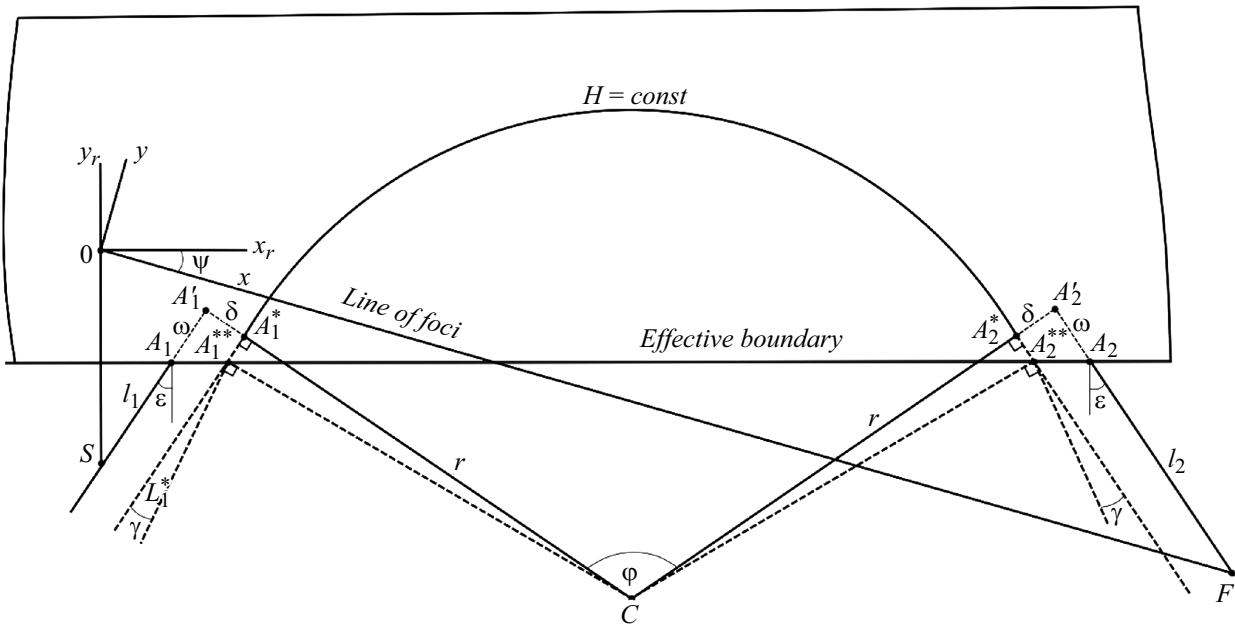
Рис. 2. Геометрическое определение положения выходного плеча l_2 оптической оси мономассового ионного пучка в масс-спектрографе на базе магнитного зеркала. Углы \epsilon и \gamma соответствуют отрицательным значениям, точки S и F отвечают положению выходной щели источника и фокусу расходящегося из точки S мономассового ионного пучка, радиус оси которого в однородном поле МЗ равен r .
