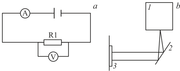
Рис. 6. Схемы измерения фототока: принципиальная электрическая схема (а), схема лазерной накачки поверхности образца: 1 — источник лазерного излучения, 2 — зеркало, 3 — образец (b).
