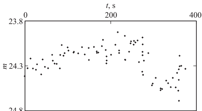
Рис. 2. Кривая блеска астероида 2023 DZ2.
