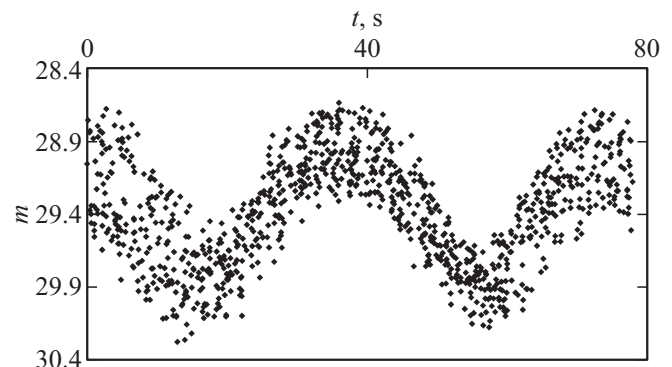
Рис. 1. Кривая блеска астероида 2023 BU, построенная по наблюдательным данным 25 января 2023 г.
