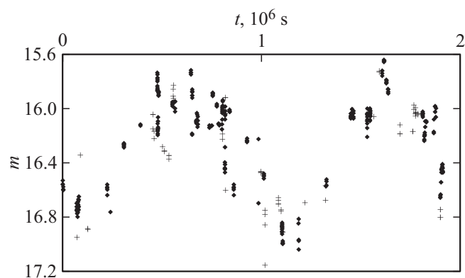
Рис. 3. Кривая блеска астероида 1998 XB.
