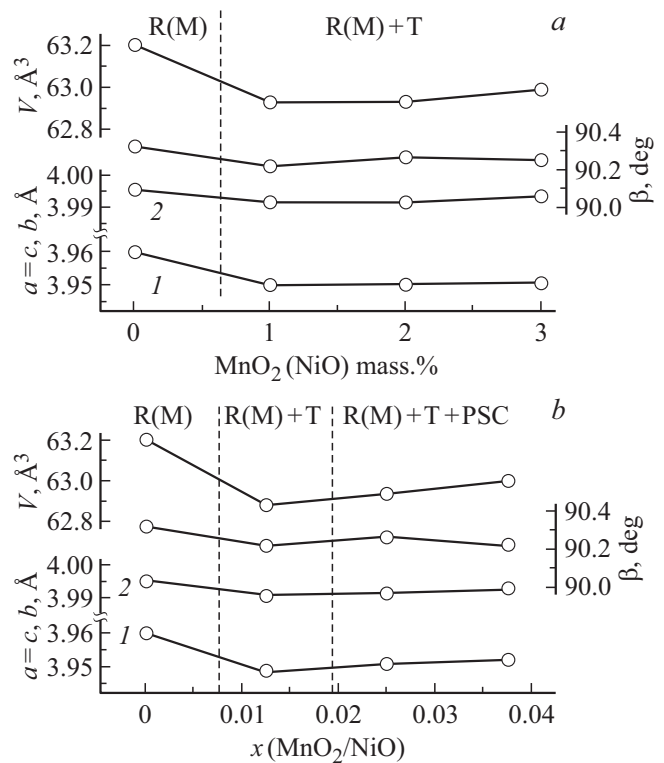
Рис. 6. Зависимости параметров перовскитной моноклинной ячейки исходного ТР с 2 \text{mass.}\% \text{NiO} , а) сверхстехиометрически и б) стехиометрически модифицированного \text{MnO}_2 от x : кривые 1 — б, 2 — а = с.
