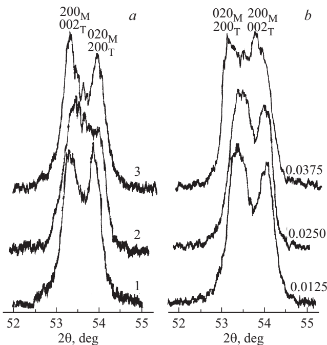
Рис. 5. Дифракционные пики (200)_c исходного ТР с оксидом \text{NiO} , а) сверхстехиометрически (числа справа — \text{mass.}\% ) и б) стехиометрически (числа справа — x ) модифицированного \text{MnO}_2 .
