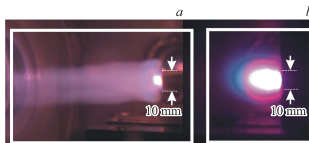
Рис. 4. Фотографии плазменных образований, экспозиция 1 с, при частоте повторения 10 Hz: а — с трубкой, б — с отверстием в графите.
