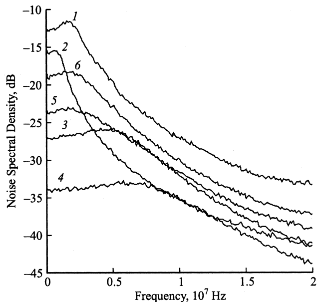
Рис. 1. Спектральная плотность шума образцов с глубиной p-n -перехода 1.33 \cdot 10^{-4} см при различных потоках облучения и температурах отжига. Поток облучения, см -2 : 1 — 0, 2 — 1.8 \cdot 10^{16} , 3 — 6.0 \cdot 10^{17} , 4 — 1.14 \cdot 10^{18} . Температура отжига, °C: 5 — 240, 6 — 340.
