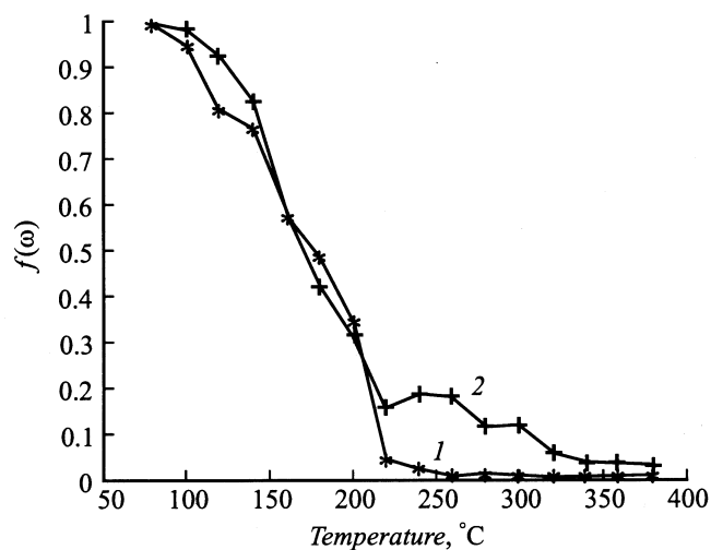
Рис. 3. Изменение ширины низкочастотного плато спектральной плотности шума при изохронном отжиге дефектов. Времена термодиффузии основного p-n -перехода, мин: 1 — 120, 2 — 75.
