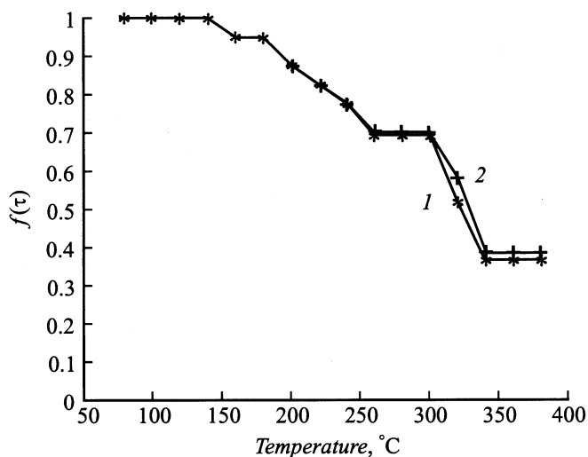
Рис. 2. Изменение эффективного времени жизни неосновных носителей заряда при изохронном отжиге дефектов. Времена термодиффузии основного p-n -перехода, мин: 1 — 120, 2 — 75.
