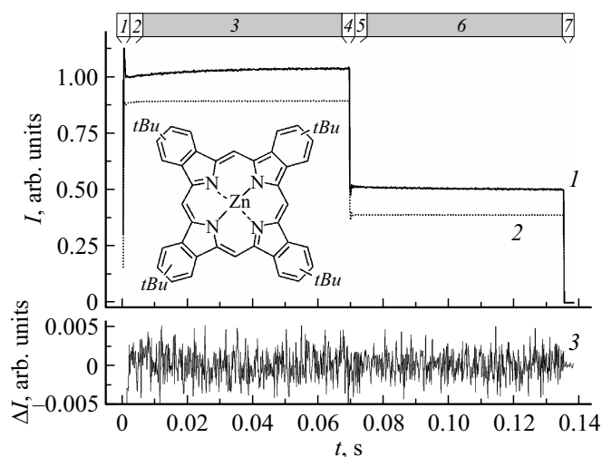
Рис. 1. Кинетика флуоресценции Zn-( tBu ) 4 -ТБП в пленке ПВБ при T = 293 \text{ K} , \lambda_{\text{det}} = 632 \text{ nm} и \lambda_{\text{exc}} = 405 \text{ nm} (кривая 1), профиль интенсивности ФВ (2), относительная разность интенсивностей экспериментальной и оптимизированной кинетических кривых (3). На вставке изображена структура Zn-( tBu ) 4 -ТБП.
