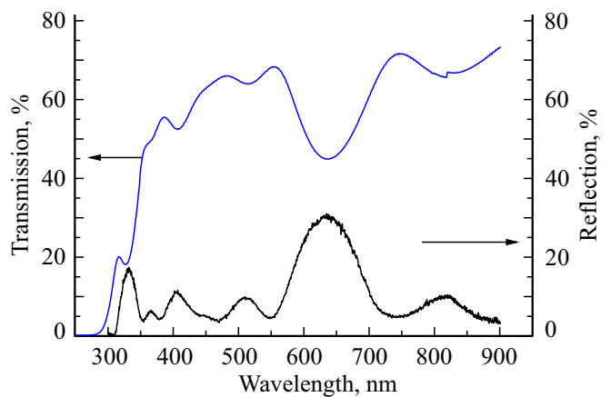
Рис. 5. Спектры оптического пропускания и отражения образца № 2 (пленки BaTiO_3/SiO_2/BaTiO_3/SiO_2/BaTiO_3 на кварце).
