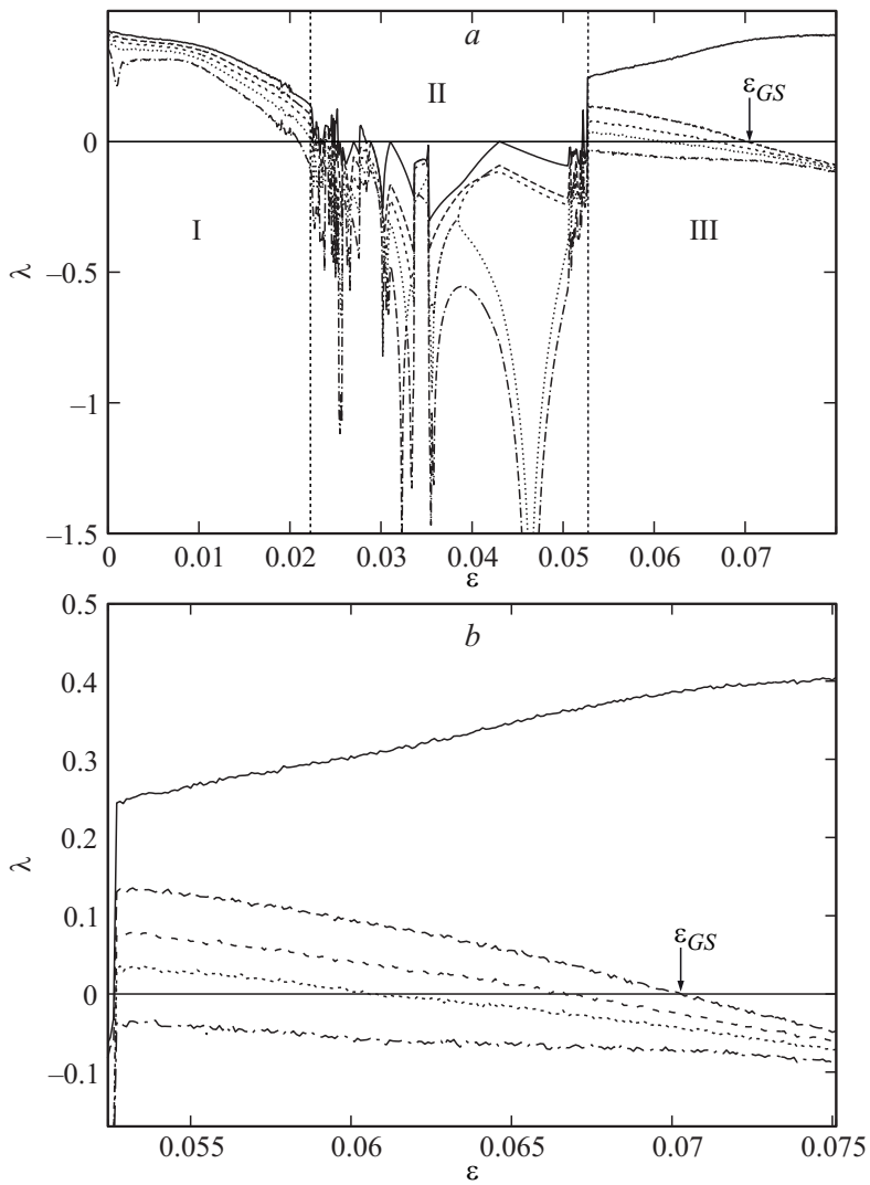
Рис. 2. a — зависимость пяти показателей Ляпунова от коэффициента связи \varepsilon , b — область значений III в более крупном масштабе.
