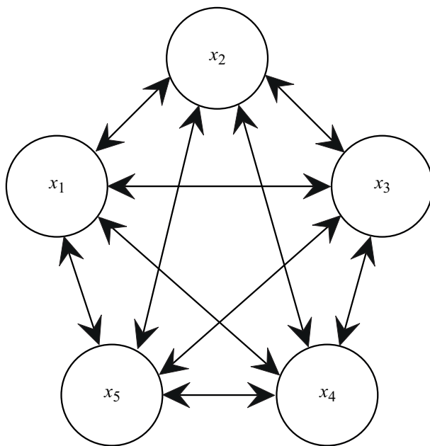
Рис. 1. Топология рассматриваемой сети из пяти логистических отображений.
