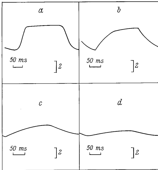
Рис. 2. Кинетика нарастания и спада стационарной ФП в облученном кремнии ( \lambda = 3.9 \mu\text{м} ) после предварительной подсветки на длине волны \lambda = 2 \mu\text{м} по прошествии после подсветки промежутка времени, с: a — 5, b — 30, c — 100, d — 500.
