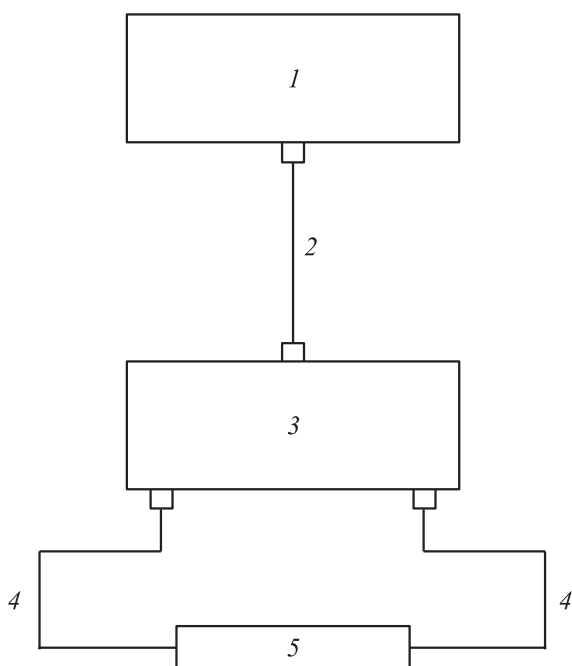
Рис. 1. Цифрами на рисунке обозначены: 1 — персональный компьютер, 2 — цифровой анализатор СВЧ-цепей, 3 — гибкий коаксиальный соединительный кабель с волновым сопротивлением 50 \Omega , 4 — коаксиальная измерительная ячейка, заполненная исследуемым веществом.
