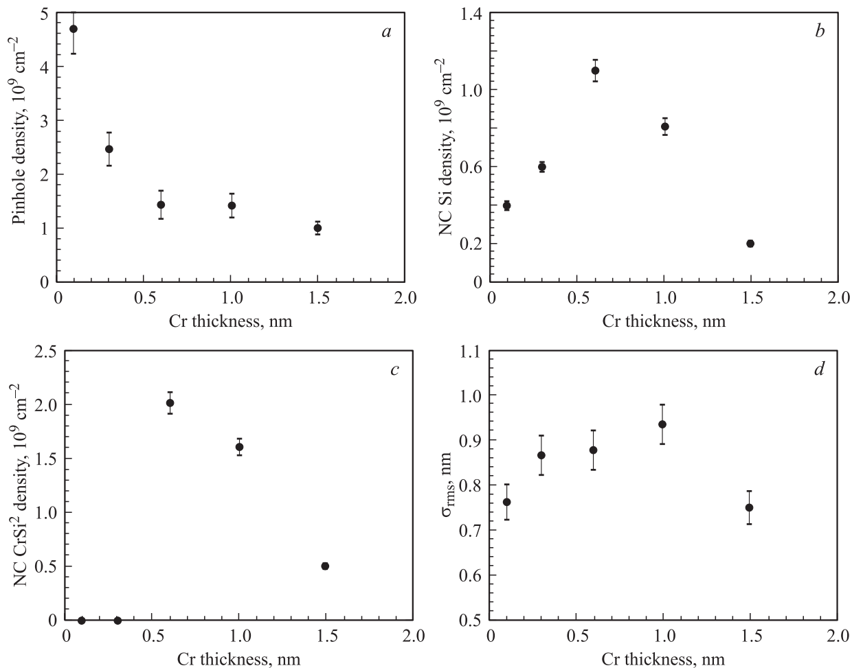
Рис. 3. Зависимости от толщины осажденного хрома плотности углублений (а), плотности кремниевых нанокристаллитов на поверхности кремния (b), плотности нанокристаллитов CrSi 2 , неполовностью встроены в углубления (с), и среднеквадратичной шероховатости ( \sigma_{\text{rms}} ) слоев кремния (d).
