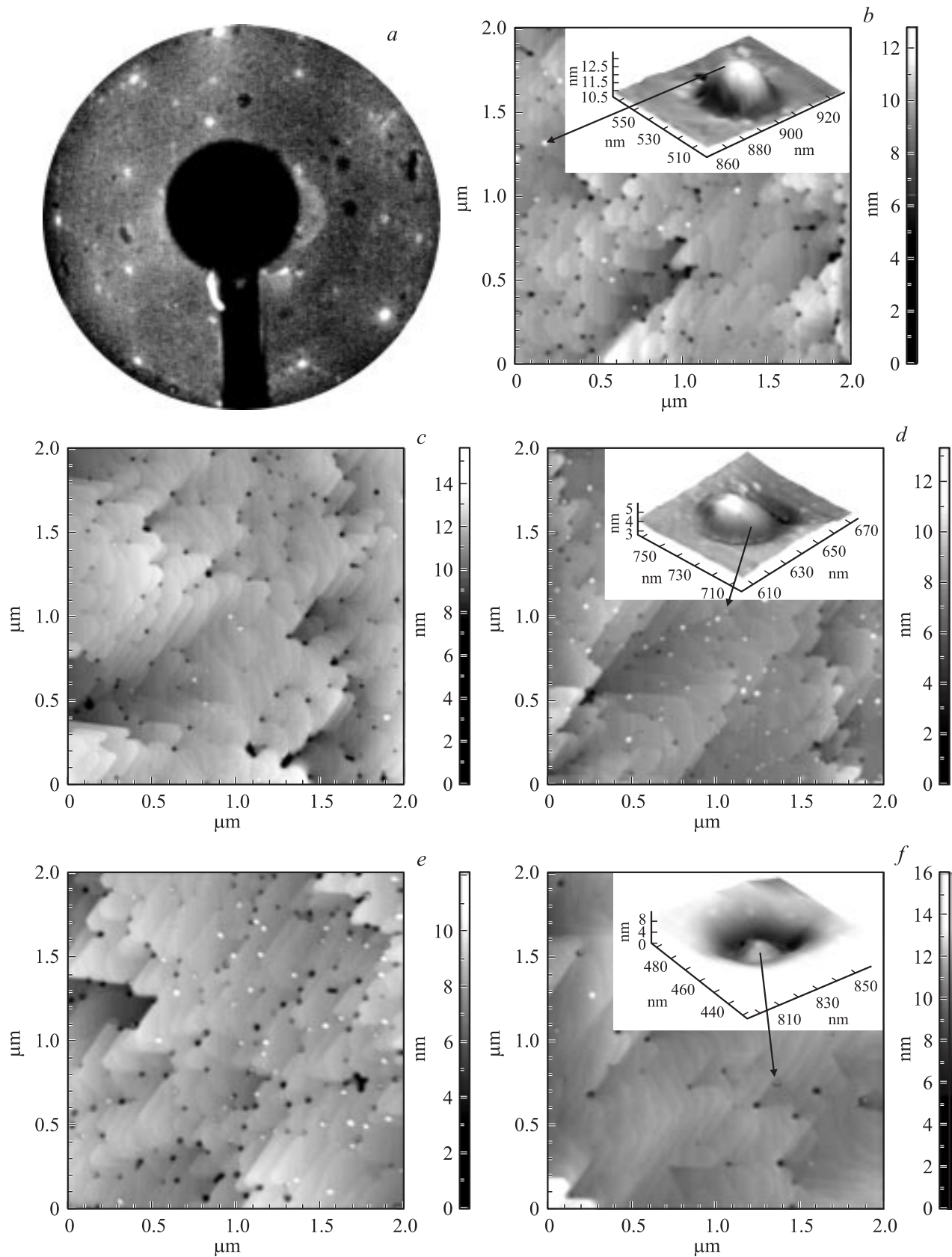
Рис. 2. Картина ДМЭ после роста кремния толщиной 100 nm поверх островков CrSi 2 ( d_{Cr} = 1.5 nm) при температуре 700°C (a) и картины АСМ для образцов с различными толщинами осажденного кремния при T = 700^\circ\text{C} поверх островков CrSi 2 на Si(100) с толщинами хрома, равными 0.1 (b), 0.3 (c), 0.6 (d), 1.0 (e) и 1.5 nm (f). На вставках изображены островок кремния (b) и невстроенные нанокристаллиты CrSi 2 (d, f).
