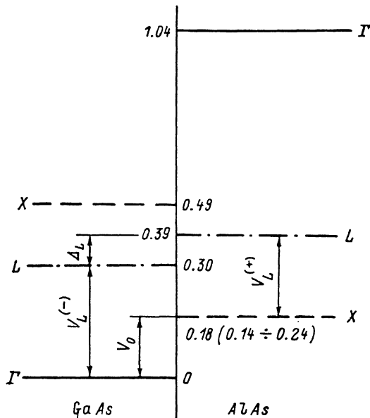
Рис. 1. Энергетическая диаграмма GaAs/AlAs-гетероперехода (цифры — энергия в эВ).
