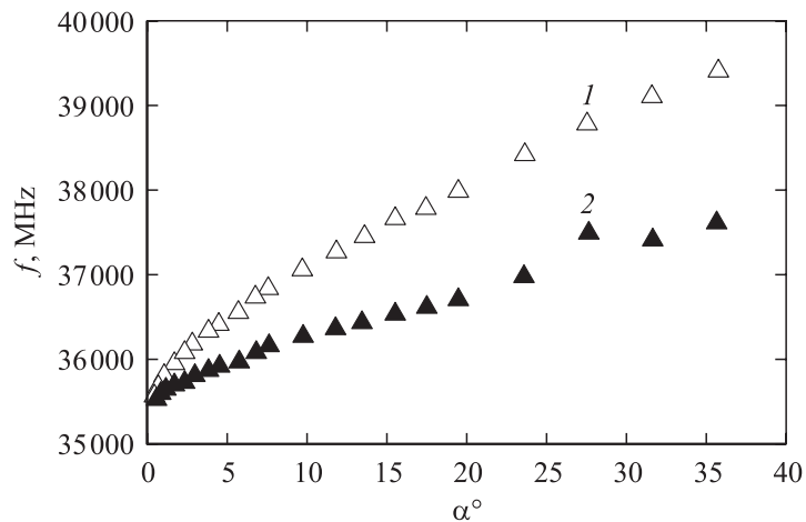
Рис. 1. Собственная частота f как функция угла наклона \alpha образующей конуса для конического квазиоптического диэлектрического резонатора: открытого (1) и с торцевой проводящей стенкой (2).
