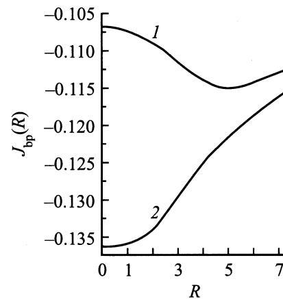
Рис. 1. Зависимость энергии биполярона от расстояния между центрами поляризонных ям без учета (1) и с учетом корреляции (2). Расчеты выполнялись для n = 5 в выражении (4).
