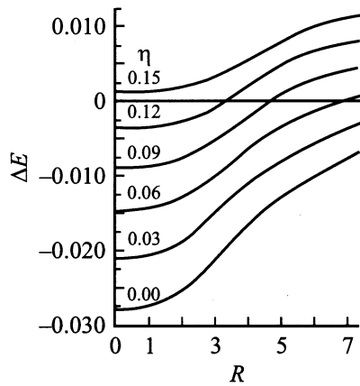
Рис. 2. Зависимость энергии связи биполярона от расстояния между центрами поляризационных ям для различных параметров ионной связи \eta . Расчеты выполнялись для n = 5 в выражении (4).
