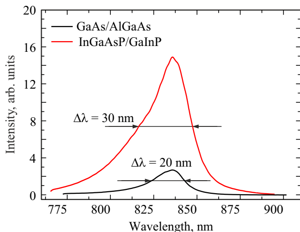
Рис. 4. Спектры фотолуминесценции Al-содержащей и без-алюминиевой ГС.
