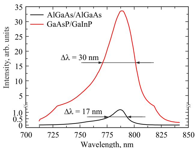
Рис. 1. Спектры фотолюминесценции Al-содержащей и безалюминиевой ГС.
