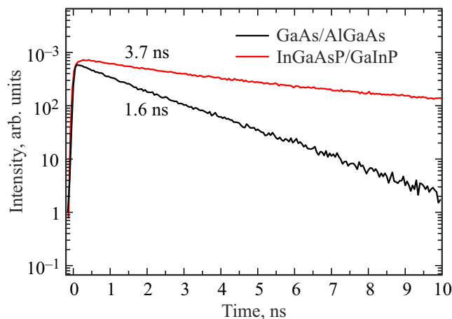
Рис. 5. Время-разрешенная фотолуминесценция квантово-размерных Al-содержащей и не содержащей Al ГС спектрального диапазона 830–850 нм.
