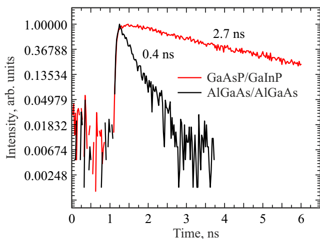
Рис. 3. Время-разрешенная фотолуминесценция квантово-размерных Al-содержащей и не содержащей Al ГС спектрального диапазона 780–800 нм.
