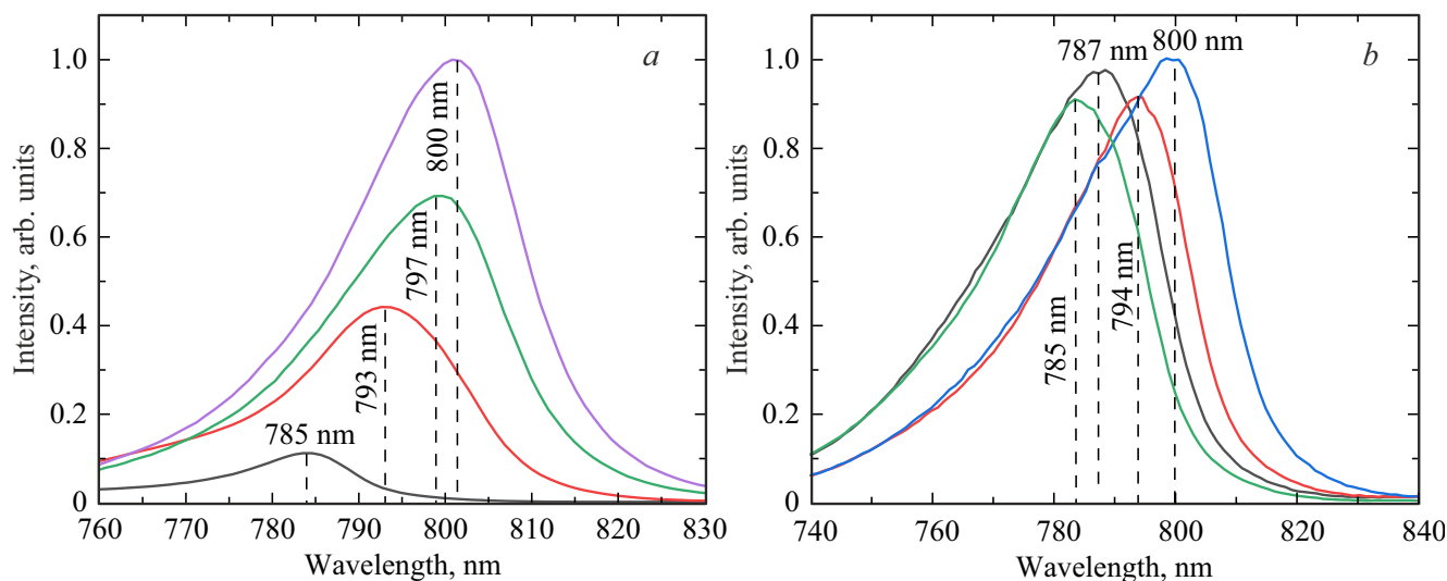
Рис. 2. Спектры фотолюминесценции Al-содержащих ( a ) и безалюминиевых ( b ) ГС гетероструктур с центральной длиной волны фотолюминесценции 780–800 нм.
