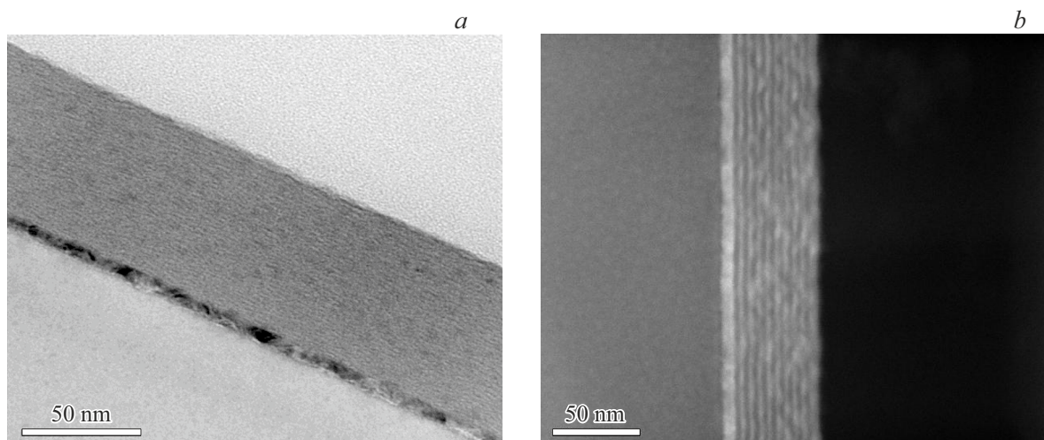
Рис. 1. a, b — ТЕМ-изображения полученных сверхрешеток GaN/InP: a — OX1132, b — OX1133.
