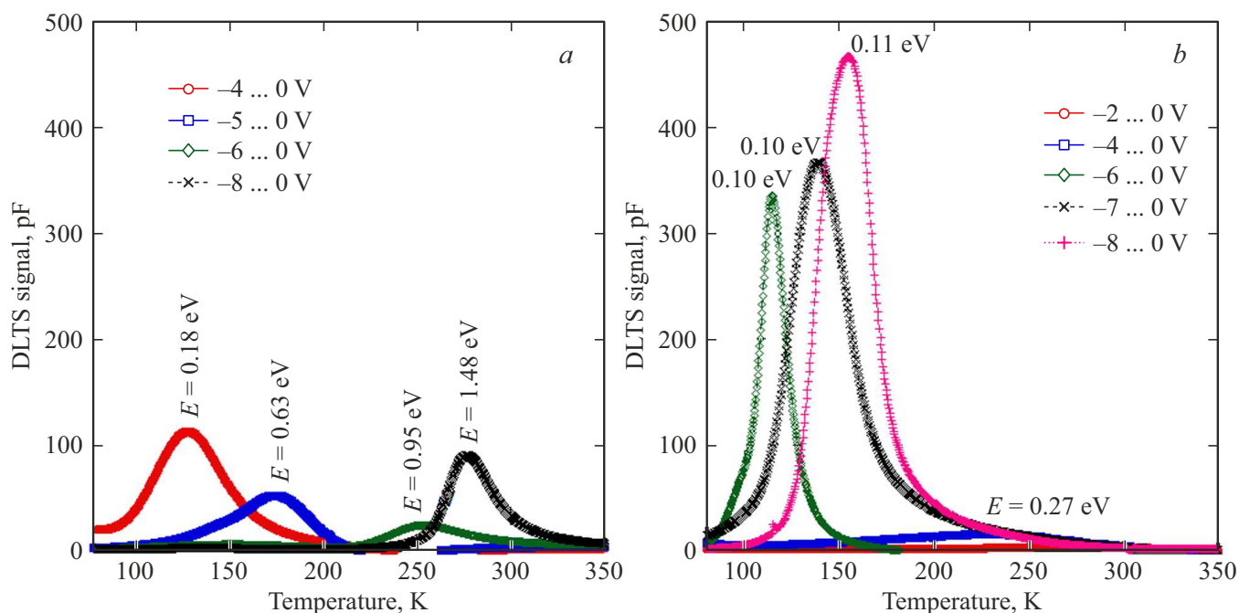
Рис. 3. a, b — график НСГУ сигнала для обоих образцов ( a — OX1132, b — OX1133) для напряжений обратного смещения от -2 до -8 В.
