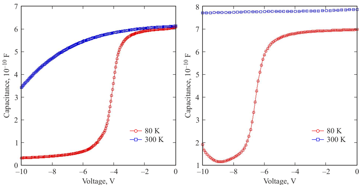
Рис. 2. a, b — вольт-фарадные характеристики образцов OX1132 ( a ) и OX1133 ( b ).
