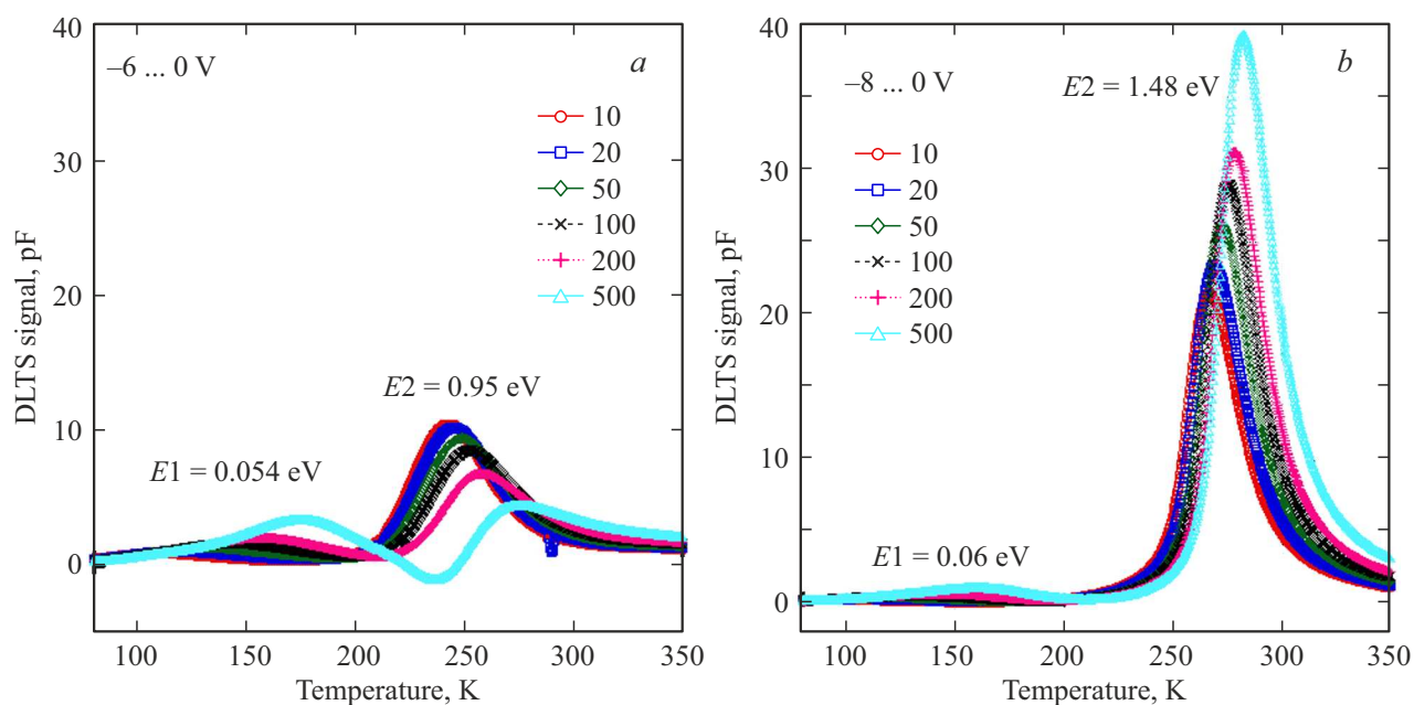
Рис. 4. a, b — график НСГУ сигнала образца OX1132, измеренный при обратных напряжениях -6-0 В ( a ) и -8-0 В ( b ) для темпов эмиссии 10, 20, 50, 100, 200, 500.
