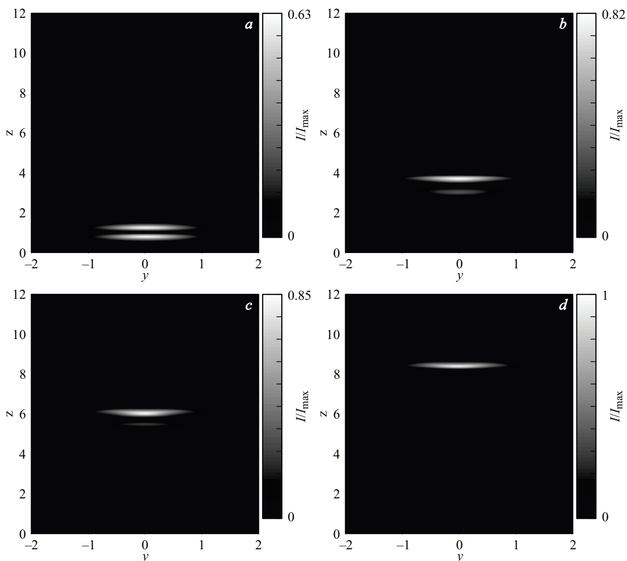
Рис. 2. Интенсивность электрического поля импульса в различные моменты времени ( n_z = 80\% , n_a = 20\% ): a — t = 0 ; b — t = 42 fs; c — t = 84 fs; d — t = 126 fs. Цветовая шкала приведена для интенсивности, отнесенной к максимуму интенсивности для всех рисунков ( a-d ).
