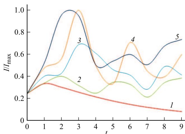
Рис. 4. Зависимость максимального значения интенсивности электромагнитного импульса от времени для разной доли УНТ типа armchair ( n_a ): 1 — n_a = 0\% ; 2 — n_a = 20\% ; 3 — n_a = 50\% ; 4 — n_a = 80\% ; 5 — n_a = 100\% . Единица по временной оси соответствует 14 fs.
