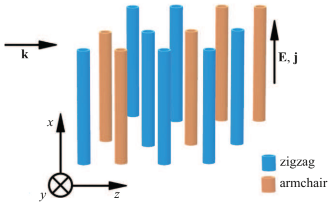
Рис. 1. Схематическое изображение геометрии системы со смешанным массивом УНТ.
