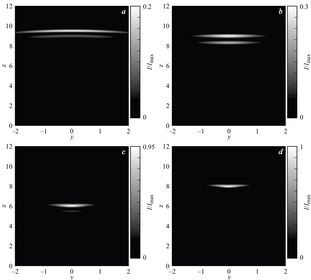
Рис. 3. Интенсивность электромагнитного импульса в момент времени t = 126 fs: a — n_z = 100\% , n_a = 0\% ; b — n_z = 90\% , n_a = 10\% ; c — n_z = 80\% , n_a = 20\% ; d — n_z = 60\% , n_a = 40\% . Цветовая шкала отображает интенсивность, приведенную к максимуму интенсивности для всех рисунков. Единица по координатным осям соответствует 4.2 \mu\text{m} .
