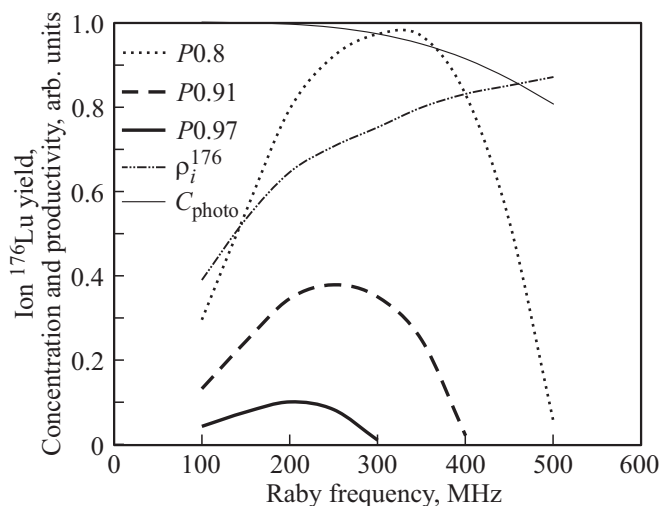
Рис. 7. Значения выхода целевого изотопа \rho_i^{176} и концентрации C_{\text{photo}} целевого изотопа ^{176}\text{Lu} при равных частотах Раби V_1 = V_2 = \gamma_i и нулевом угле \theta отклонения атомов (штрихпунктирная и тонкая линии соответственно). Расчет производительности с заданной концентрацией целевого изотопа ^{176}\text{Lu} C_p = 0.8; 0.91; 0.97 в зависимости от частоты Раби, с использованием выражений (22) и (23) для производительности продукта с заданной концентрацией целевого изотопа C_p (пунктирная, штриховая и сплошная толстая линии).
