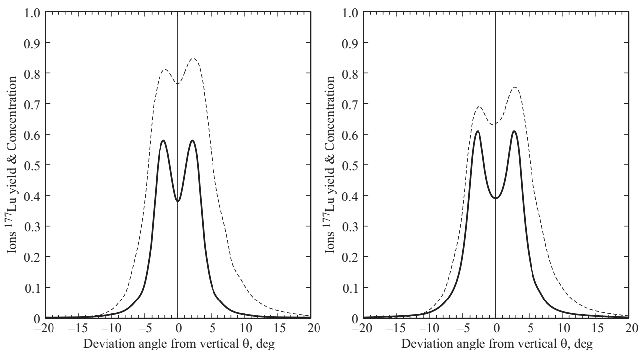
Рис. 9. Результаты расчета зависимости относительного выхода целевого изотопа ^{177}\text{Lu} (сплошные линии) и его концентрации в ансамбле фотоионов C_{\text{photo}} (пунктирные линии) при фотоионизации облученной в реакторе природной смеси с начальной концентрацией ^{177}\text{Lu} 3.4 \cdot 10^{-5} от угла отклонения \theta . Слева — при частотах Раби V_1 = 40 \text{ MHz} , V_2 = 126 \text{ MHz} , \gamma_i = 255 \cdot 10^6 \text{ 1/s} . Справа — при частотах Раби V_1 = 47 \text{ MHz} , V_2 = 150 \text{ MHz} , \gamma_i = 255 \cdot 10^6 \text{ 1/s} .
