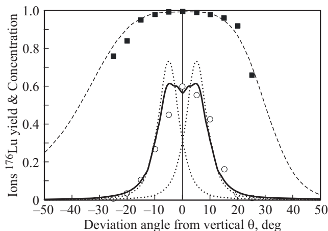
Рис. 4. Сравнение с расчетом экспериментальной зависимости относительного выхода целевого изотопа ^{176}\text{Lu} (светлые кружки) и его концентрации в ансамбле фотоионов C_{\text{photo}} (темные квадраты) от угла отклонения \theta при средних плотностях мощности лазерного излучения на первом, втором и третьем переходах P_1 = 35 \text{ mW/cm}^2 , P_2 = 22 \text{ mW/cm}^2 и P_3 = 2.25 \text{ W/cm}^2 соответственно. Расчет при частотах Раби V_1 = 129 \text{ MHz} , V_2 = 306 \text{ MHz} и скорости фотоионизации \gamma_i = 270 \text{ MHz} . Пунктиром показаны сдвинутые по углу на \pm 5^\circ результаты при V_1 = V_2 = 129 \text{ MHz} .
