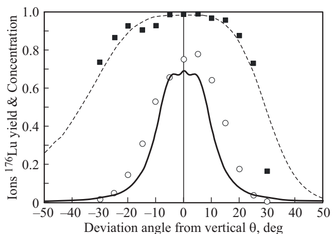
Рис. 5. Сравнение с расчетом экспериментальной зависимости относительного выхода целевого изотопа ^{176}\text{Lu} (светлые кружки) и его концентрации в ансамбле фотоионов C_{\text{photo}} (темные квадраты) от угла отклонения \theta при средних плотностях мощности лазерного излучения на первом, втором и третьем переходах P_1 = 68 \text{ mW/cm}^2 , P_2 = 26 \text{ mW/cm}^2 и P_3 = 2.25 \text{ W/cm}^2 соответственно. Расчет при частотах Раби V_1 = 180 \text{ MHz} , V_2 = 332 \text{ MHz} и скорости фотоионизации \gamma_i = 270 \text{ MHz} .
