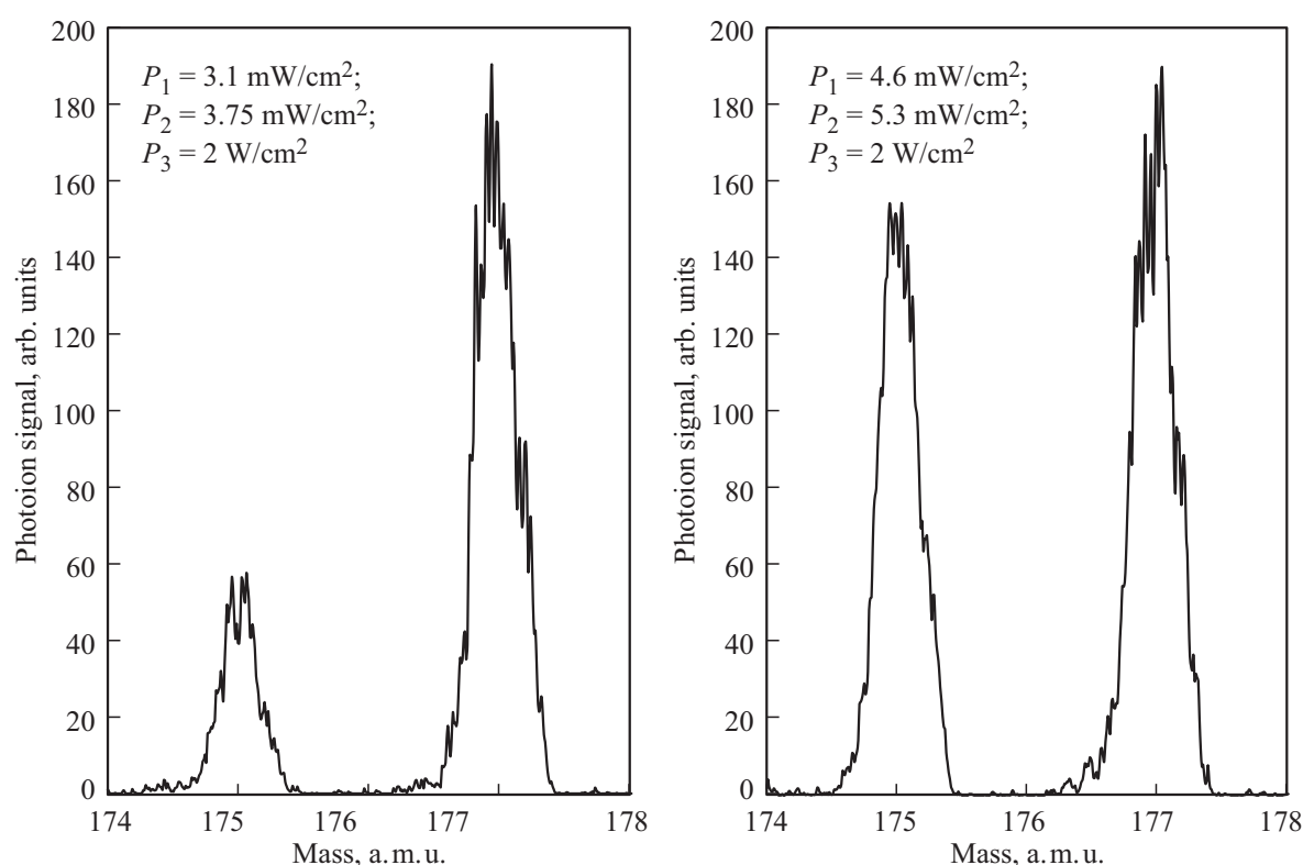
Рис. 8. Масс-спектры фотоионизации ^{177}\text{Lu} по каналу 5-6-5-4 в совмещенных импульсах при различных средних плотностях мощности лазерного излучения на первой и второй ступенях. Слева — средняя плотность мощности на первой и второй ступенях 3.1 \text{ mW/cm}^2 и 3.75 \text{ mW/cm}^2 соответственно, концентрация ^{177}\text{Lu} 73 %. Справа средняя плотность мощности на первой и второй ступенях 4.6 \text{ mW/cm}^2 и 5.3 \text{ mW/cm}^2 соответственно, концентрация ^{177}\text{Lu} 54 %. Исходная концентрация ^{177}\text{Lu} — (3.4 \pm 0.4) \cdot 10^{-5} .
