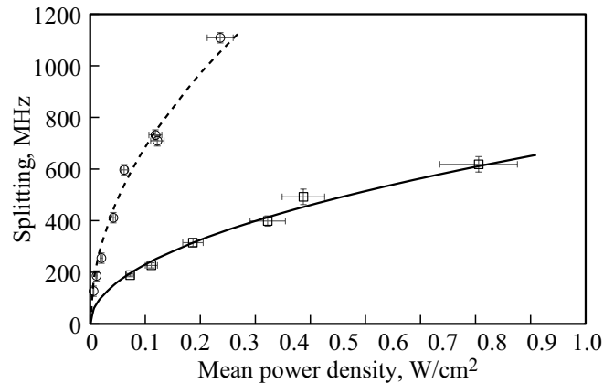
Рис. 2. Зависимость расщепления перехода от средней плотности мощности лазерного излучения [9]. Квадраты и сплошная линия — первый переход. Круги и пунктирная линия — второй переход.
