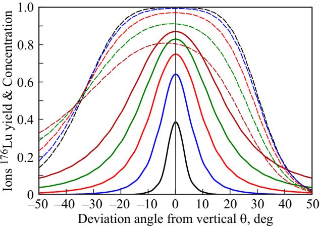
Рис. 6. Результаты расчета зависимости относительного выхода целевого изотопа 176 Lu (сплошные линии, снизу вверх от 100 до 500 МГц) и его концентрации в ансамбле фотоионов C_{photo} (штриховые линии, сверху вниз от 100 до 500 МГц) от угла отклонения \theta при частотах Раби V_1 = V_2 = 100 МГц (черные линии), 200 МГц (синие линии), 300 МГц (красные линии), 400 МГц (зеленые линии) и 500 МГц (коричневые линии) при соответствующих скоростях фотоионизации: \gamma_i = 100 \cdot 10^6 1/s, 200 \cdot 10^6 1/s, 300 \cdot 10^6 1/s, 400 \cdot 10^6 1/s, 500 \cdot 10^6 1/s.
