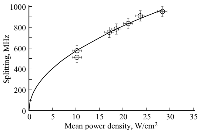
Рис. 3. Зависимость расщепления третьего перехода от средней плотности мощности лазерного излучения [4].
