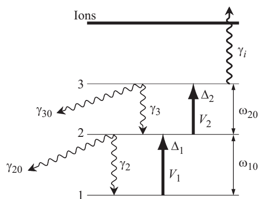
Рис. 1. Упрощенная схема трехступенчатой ионизации атома лютеция, соответствующая расчетной модели и уравнениям (2)–(8).
