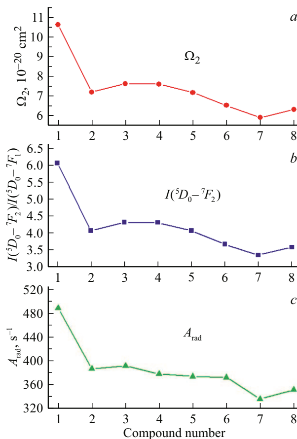
Рис. 4. Изменения параметра интенсивности \Omega_2 ( a ), относительной интенсивности I({}^5D_0-{}^7F_2)/I({}^5D_0-{}^7F_1) ( b ) и скорости излучательных процессов A_{\text{rad}} ( c ) в серии соединений 1–8 .
