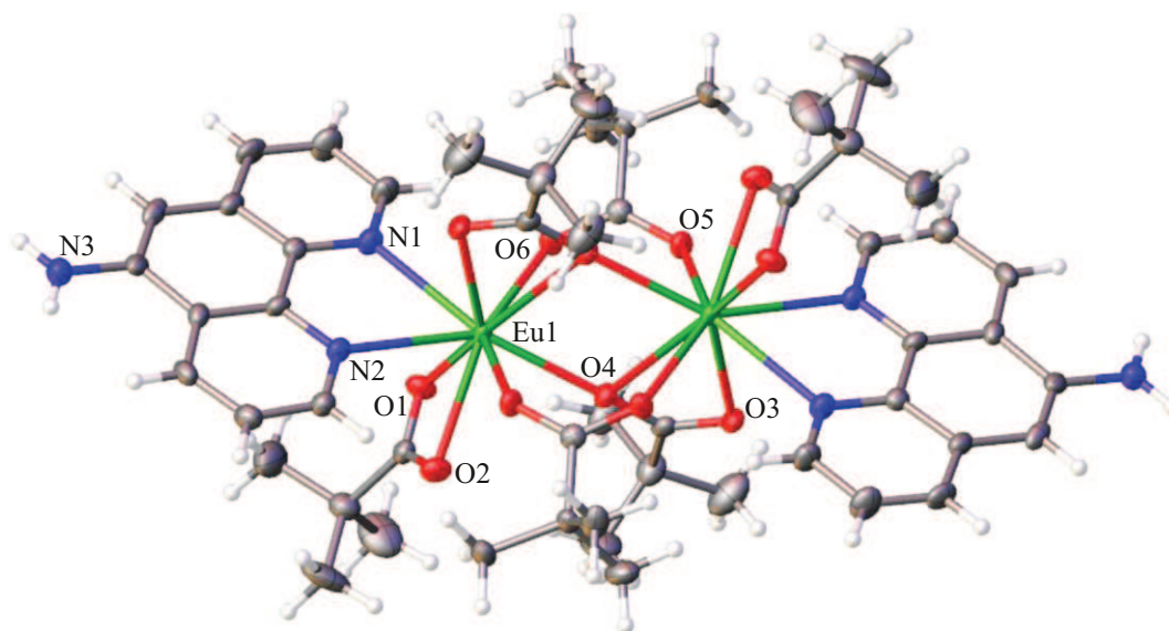
Рис. 1. Молекулярная структура димера пивалата [\text{Eu}_2(\text{Piv})_6(\text{APhen})_2] ( 4 ).
