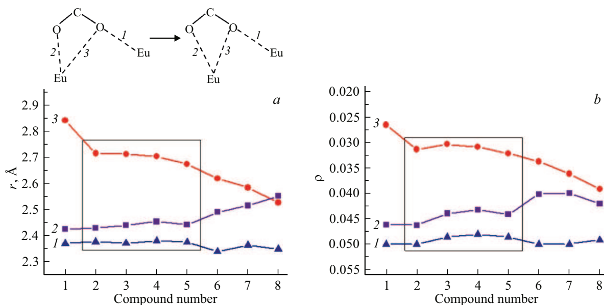
Рис. 2. Изменения длин трех связей (пронумерованы как 1, 2, 3) Eu–O r (a) и Eu–O-перекрывания \rho (b), относящиеся к мостиково-циклической группе -\text{COO}^- в серии соединений 1–8.
