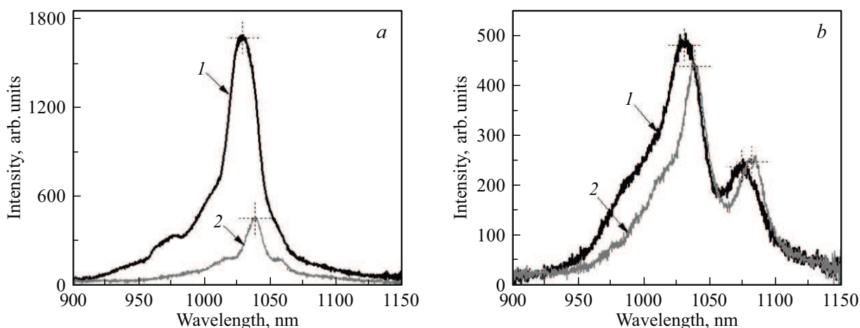
Рис. 5. Спектры люминесценции керамики \text{Yb:YAG} (a) и \text{Yb:Y}_2\text{O}_3\text{-Zr} (b), зарегистрированные непосредственно после облучения электронами (1) и спустя 1 min (2).
