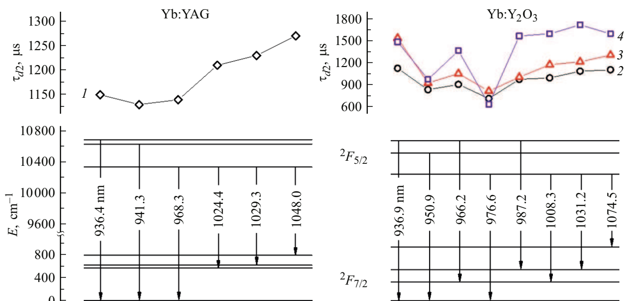
Рис. 4. Оптические переходы иона \text{Yb}^{3+} в решетке иттрий-алюминиевого граната и кубического оксида иттрия и характерные времена затухания \tau_{d2} , измеренные на соответствующих им длинах волн в керамиках \text{Yb:YAG} (1), \text{Yb:Y}_2\text{O}_3\text{-X} (2), \text{Yb:Y}_2\text{O}_3\text{-ГИП} (3) и \text{Yb:Y}_2\text{O}_3\text{-Zr} (4).
