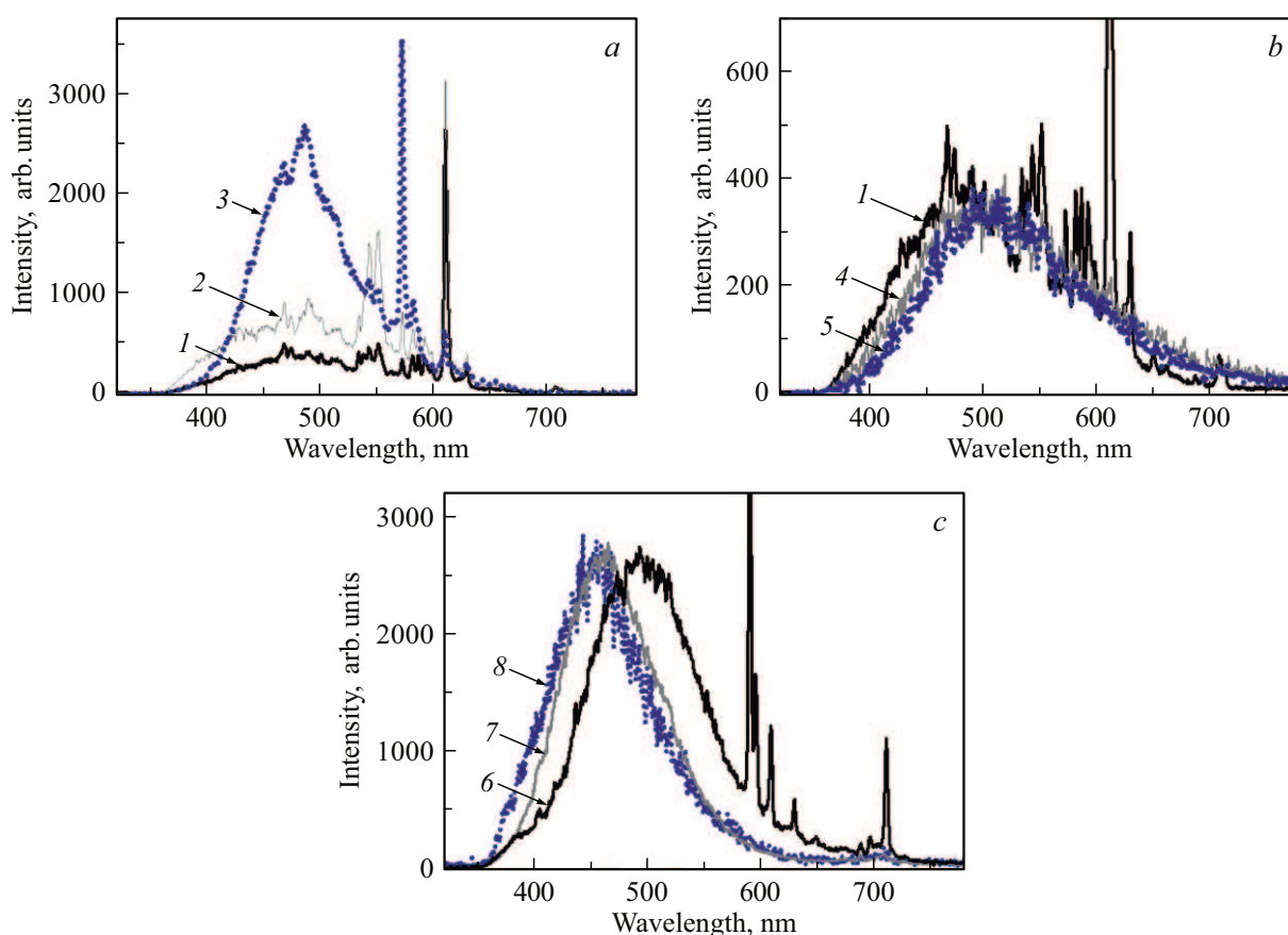
Рис. 2. Обзорные спектры ИКЛ керамических образцов активированного иттербием и „чистого“ оксида иттрия и иттрий-алюминиевого граната в видимой области спектра: a — образцы без добавления \text{ZrO}_2 : \text{Yb}:\text{Y}_2\text{O}_3\text{-X} (кривая 1), \text{Yb}:\text{Y}_2\text{O}_3\text{-ГИП} (кривая 2) и \text{Y}_2\text{O}_3 (кривая 3); b — образцы с добавлением \text{ZrO}_2 : \text{Yb}:\text{Y}_2\text{O}_3\text{-Zr} (кривая 4) и \text{Y}_2\text{O}_3\text{-Zr} (кривая 5), а также \text{Yb}:\text{Y}_2\text{O}_3\text{-X} (кривая 1) для сравнения; c — образцы \text{Yb}:\text{YAG} (кривая 6) и \text{YAG} (кривая 7 — спектр, зарегистрированный во время облучения; кривая 8 — спектр фосфоресценции, зарегистрированный через 5 s после облучения). Спектры на рисунке b и c нормированы по максимуму широкой полосы.
