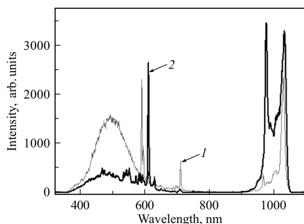
Рис. 1. Обзорные спектры импульсной катодолюминесценции керамических образцов Yb:YAG (1) и Yb:Y 2 O 3 -X (2).
