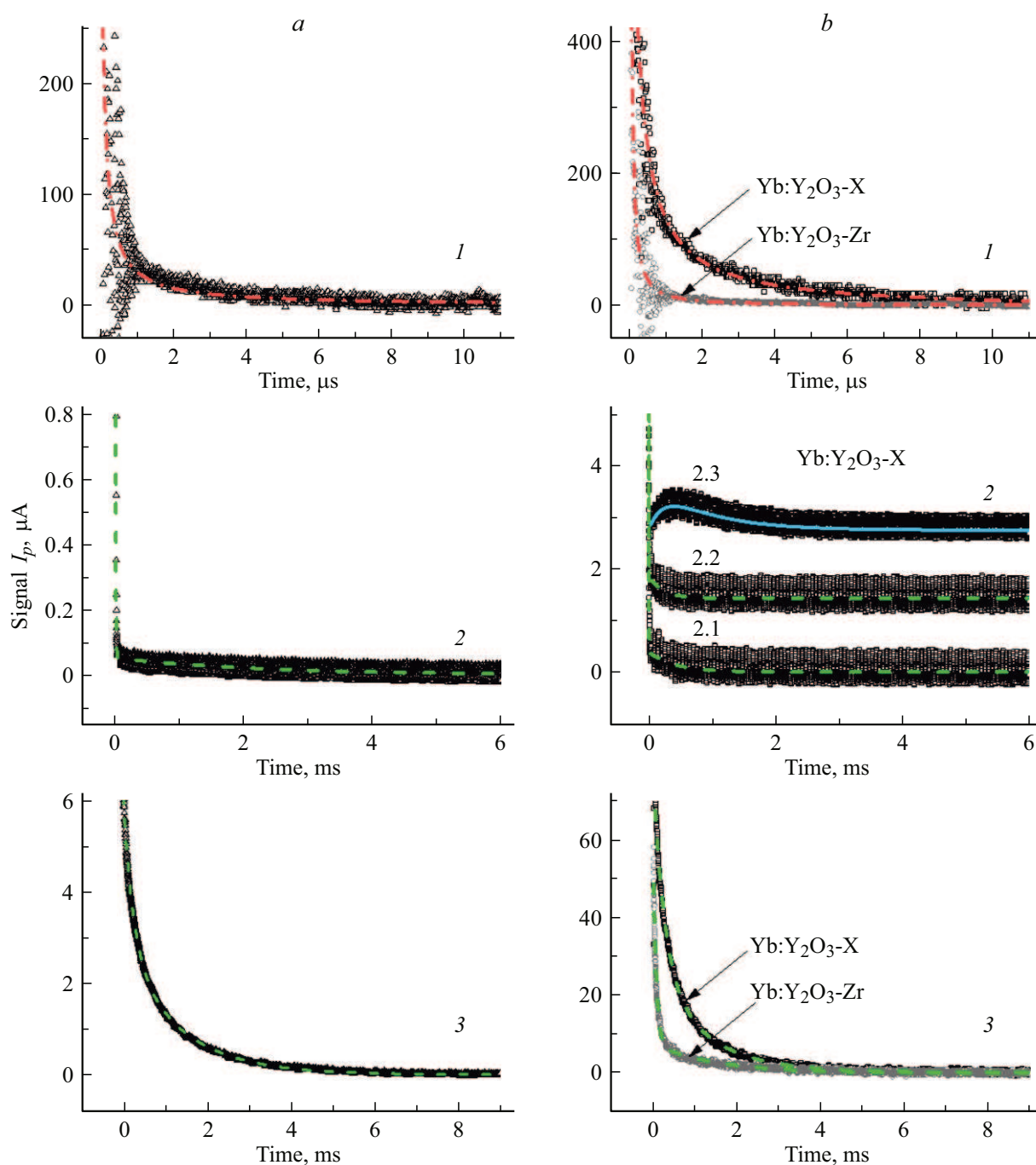
Рис. 3. Характерная кинетика люминесценции на спектральных полосах образцов (a) Yb:YAG ( I — измерение при 460 nm на коротковолновом плече полосы при 495 nm, 2 — линия при 591.0 nm и 3 — линия при 1029.3 nm) и (b) Yb:Y 2 O 3 -X и Yb:Y 2 O 3 -Zr ( I — измерение при 425 nm на коротковолновом плече широкой полосы, 2 — спектральные линии центров при 551.1 (кривая 2.1), 572.5 (кривые 2.2) и 611.0 nm (кривая 2.3), 3 — полоса при 1031.2 nm). Цветными линиями показан результат аппроксимации экспериментальных кривых: штрих-пунктирной розовой — функцией (3), штриховой зеленой — функцией (4) и сплошной синей — функцией (5).
