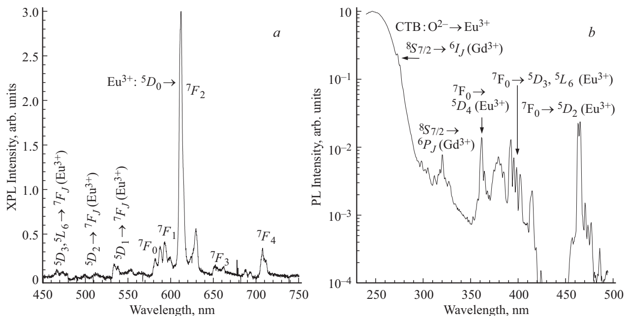
Рис. 8. Монокристалл \text{Gd}_2\text{O}_3:\text{Eu}^{3+},\text{Ce}^{3+} : (a) спектр РЛ, (b) спектр ВФЛ ( \lambda_{\text{emis}} = 611 \text{ nm} ), T = 295 \text{ K} .
