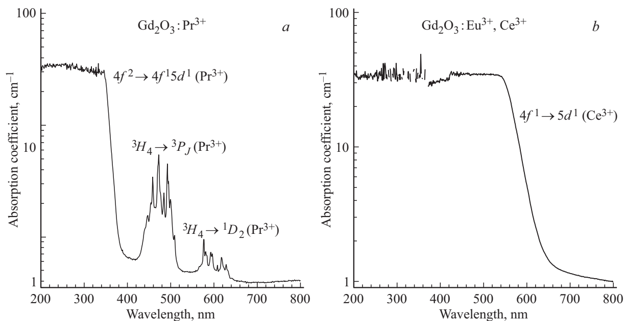
Рис. 6. Спектры поглощения монокристаллов (а) Gd_2O_3:Pr^{3+} и (b) Gd_2O_3:Eu^{3+}, Ce^{3+} .
