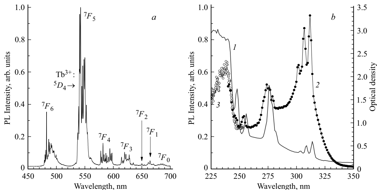
Рис. 3. Монокристалл \text{Gd}_2\text{O}_3:\text{Tb}^{3+} . (а) Спектр ФЛ ( \lambda_{\text{exc}} = 248 nm); (б) оптическая плотность (1) и спектры ВФЛ ( \lambda_{\text{emis}} = 542 nm), измеренные с применением ксеноновой (2) и дейтериевой (3) ламп, T = 295 К. Спектральное разрешение 0.2 (а) и 2 nm (б).
