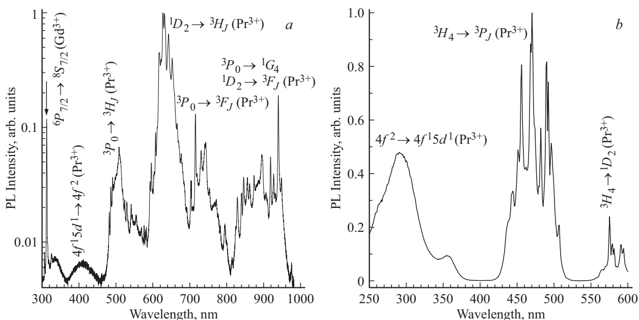
Рис. 7. Монокристалл Gd_2O_3:Pr^{3+} : (а) спектр ФЛ ( \lambda_{exc} = 272 nm), (b) спектр ВФЛ ( \lambda_{emis} = 625 nm), T = 295 K.
