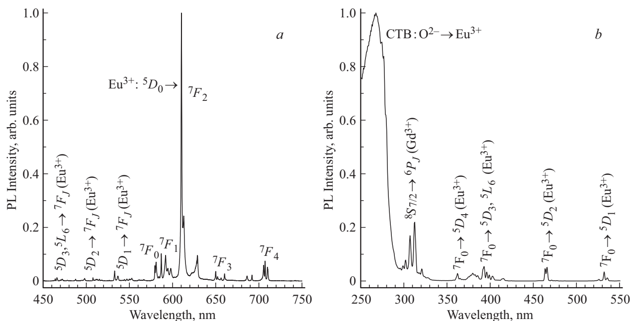
Рис. 4. Монокристалл Gd_2O_3:Eu^{3+} . (а) Спектр ФЛ ( \lambda_{exc} = 270 nm); (б) спектр ВФЛ ( \lambda_{emis} = 611 nm), T = 295 K.
