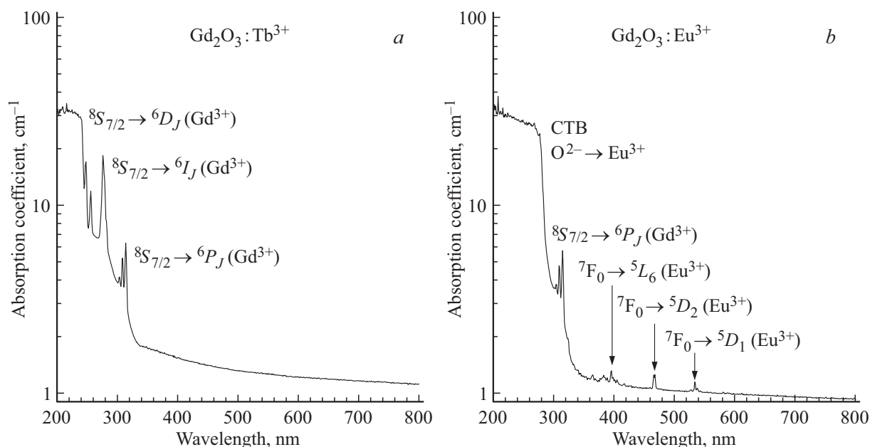
Рис. 2. Спектры поглощения монокристаллов (а) Gd_2O_3:Tb^{3+} и (б) Gd_2O_3:Eu^{3+} .
