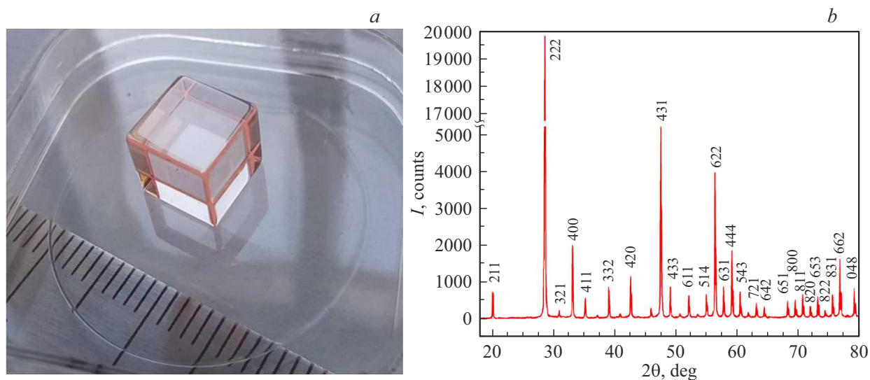
Рис. 1. (а) Фотография выращенного монокристалла \text{Gd}_2\text{O}_3:\text{Eu}^{3+} , (b) порошковая рентгеновская дифрактограмма монокристалла \text{Gd}_2\text{O}_3:\text{Eu}^{3+} .
