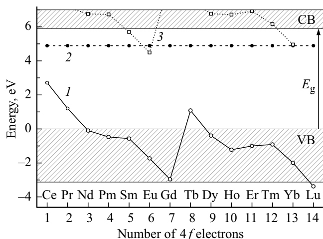
Рис. 5. Рассчитанная диаграмма энергетических уровней лантаноидов в Gd_2O_3 в зависимости от количества электронов в основном состоянии 4f^n -конфигурации трехвалентного иона лантаноида [16]. Кривые 1 и 2 соответствуют низшим уровням 4f^n - и 4f^{n-1}5d^1 -конфигураций трехвалентных лантаноидов соответственно. Кривая 3 соответствует нижним уровням 4f^{n+1} -конфигурации двухвалентных лантаноидов.
