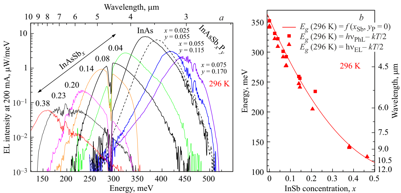
Рис. 2. Спектры ЭЛ p - n -гетероструктур с активными областями, содержащими \text{InAs}_{1-x}\text{Sb}_x ( x \leq 0.38 ), \text{InAs} , \text{InAs}_{1-x-y}\text{Sb}_x\text{P}_y ( y \approx 2.2x , x \leq 0.075 ) (a), значения энергий, соответствующих ширине запрещенной зоны активной области, полученные из данных по фото- и электролюминесценции (b) при T = 296 K.
