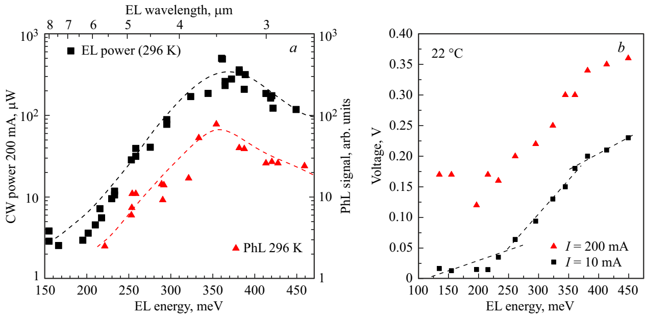
Рис. 3. Зависимости мощности ЭЛ и интенсивности ФЛ p - n -гетероструктур (a) и напряжения при токе накачки 10 и 200 мА (b) от энергии в максимуме излучения ( T = 296 \text{ K} ).
