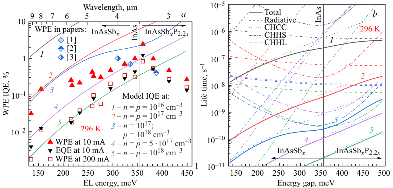
Рис. 4. Зависимости КПД (WPE) при токе накачки 10 и 200 мА, EQE при токе накачки 10 мА и расчетных значений внутренней квантовой эффективности от энергии в максимуме излучения (a) и расчетные значения времен жизни для излучательной и оже-рекомбинаций (b) при комнатной температуре при различных уровнях инжекции (указанных на фрагменте a).
