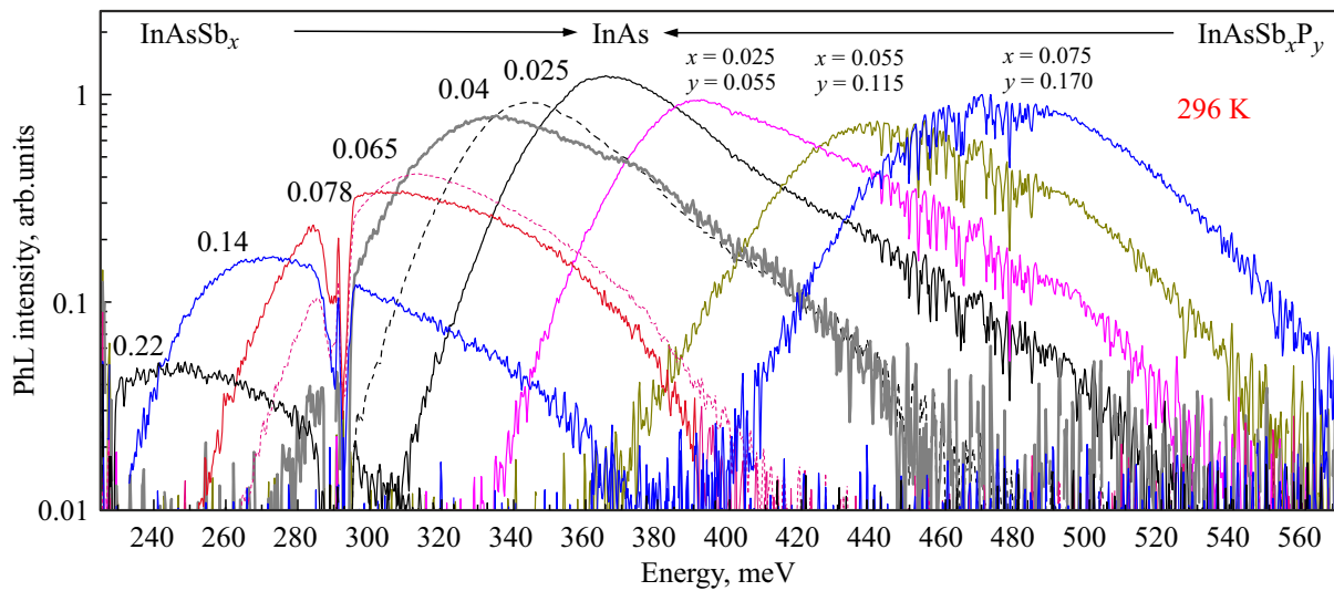
Рис. 1. Спектры ФЛ p - n -гетероструктур с активными областями, содержащими \text{InAs}_{1-x}\text{Sb}_x ( x \leq 0.22 ), \text{InAs} , \text{InAs}_{1-x-y}\text{Sb}_x\text{P}_y ( y \approx 2.2x , x \leq 0.075 ) при T = 296 K.
