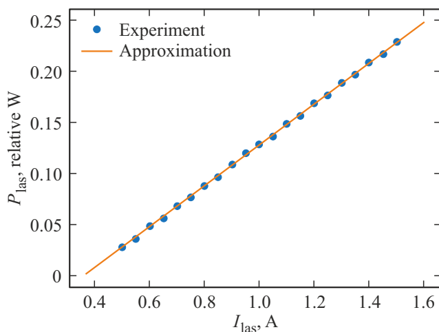
Рис. 1. Зависимость оптической мощности лазера, используемого в экспериментах, от тока, пропускаемого через него.
