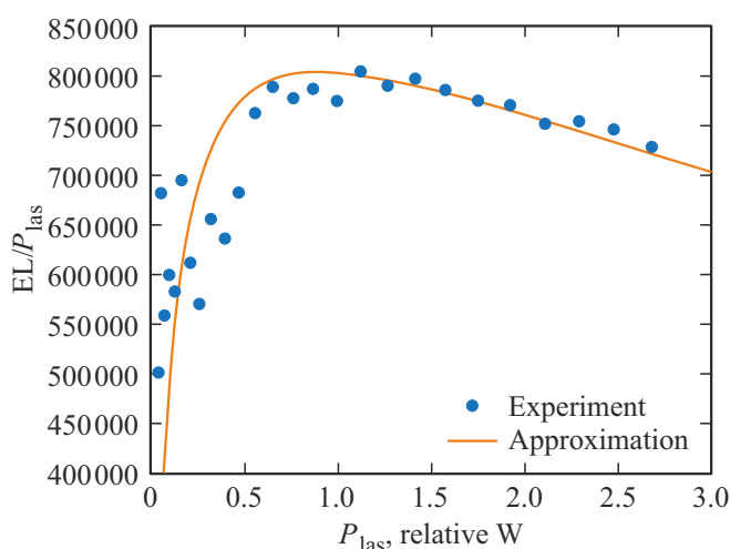
Рис. 4. Экспериментальная зависимость отношения интенсивности ЭЛ ( L ) к мощности лазерного излучения ( P_{\text{las}} ) от мощности лазерного излучения (символы), а также результат аппроксимации с использованием выражения (4) этой зависимости (линия).
