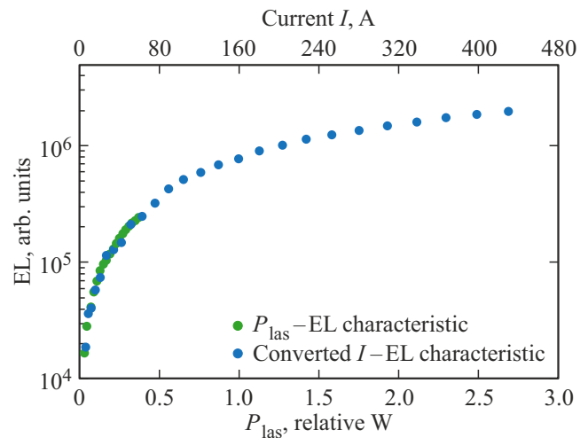
Рис. 2. Экспериментальная зависимость интенсивности ЭЛ ( L ) от мощности лазера ( P_{las} ): зеленые точки — область, где нет перегрева контрольного образца СИД лазерным излучением.
