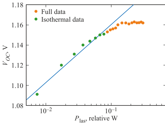
Рис. 3. Зависимость напряжения холостого хода ( V_{OC} ) контрольного образца СИД от мощности лазерного излучения ( P_{las} ): зеленые точки — область, где зависимость подчиняется уравнению (3), оранжевые точки — область перегрева контрольного образца СИД лазерным излучением.
